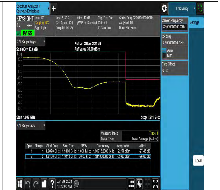
Band2_3MHz_QPSK_19185_1RB#0
