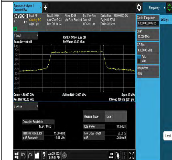
Band2-20MHz-QPSK-18900-100RB#0-PASS
