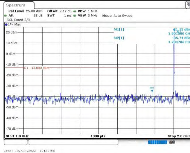
Band2-10MHz-16QAM-19150-1RB#0-Range2:1000~2000MHz
