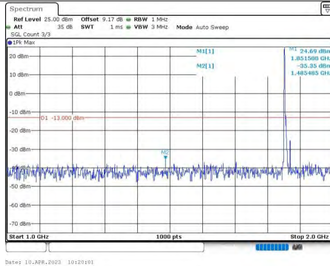
Band2-10MHz-QPSK-18650-1RB#0-Range2:1000~2000MHz
