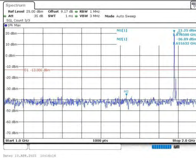
Band2-5MHz-QPSK-18900-1RB#0-Range2:1000~2000MHz
