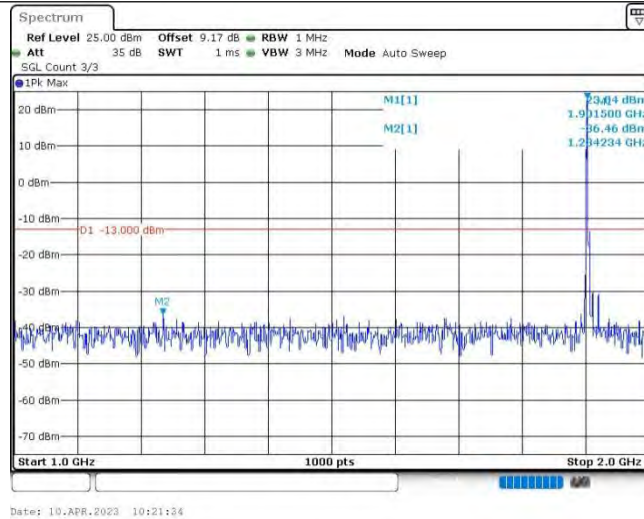
Band2-10MHz-QPSK-19150-1RB#0-Range2:1000~2000MHz
