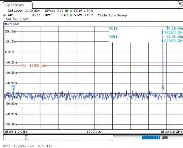
Band2-3MHz-QPSK-18900-1RB#0-Range2:1000~2000MHz
