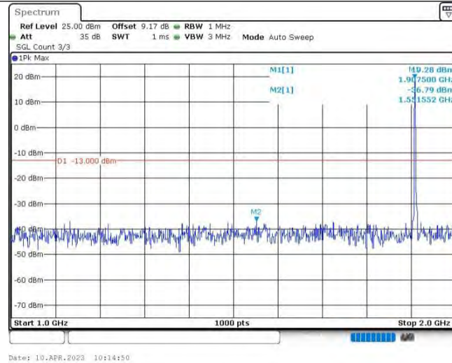
Band2-3MHz-16QAM-19185-1RB#0-Range2:1000~2000MHz
