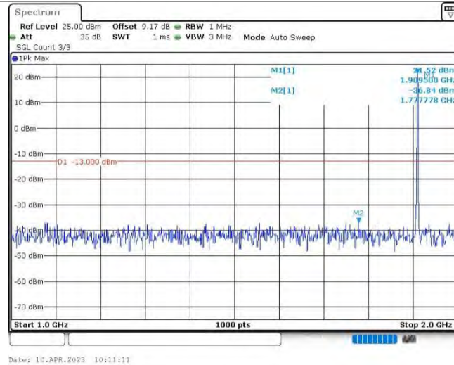
Band2-1.4MHz-QPSK-19193-1RB#0-Range2:1000~2000MHz
