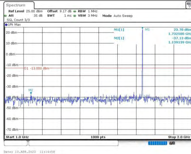
Band4-1.4MHz-QPSK-20175-1RB#0-Range2:1000~2000MHz
