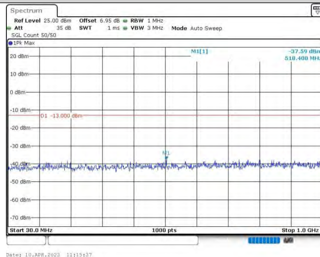
Band4-1.4MHz-QPSK-20393-1RB#0-Range1:30~1000MHz
