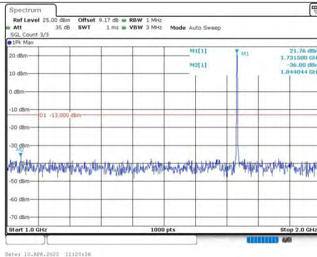
Band4-3MHz-QPSK-20175-1RB#0-Range2:1000~2000MHz
