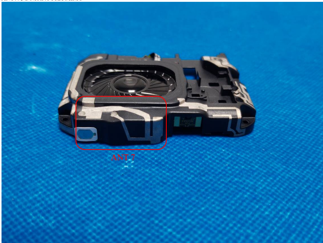
ANT4: GSM850/PCS1900, WCDMA B2/B4/B5, LTE B2/4/5/7/12/13/17/26/38/40/41/66, 5G NR n2/5/7/26/38/66 DRX MIMO ANT5: No use ANT7: 5G NR n41 PRX MIMO
