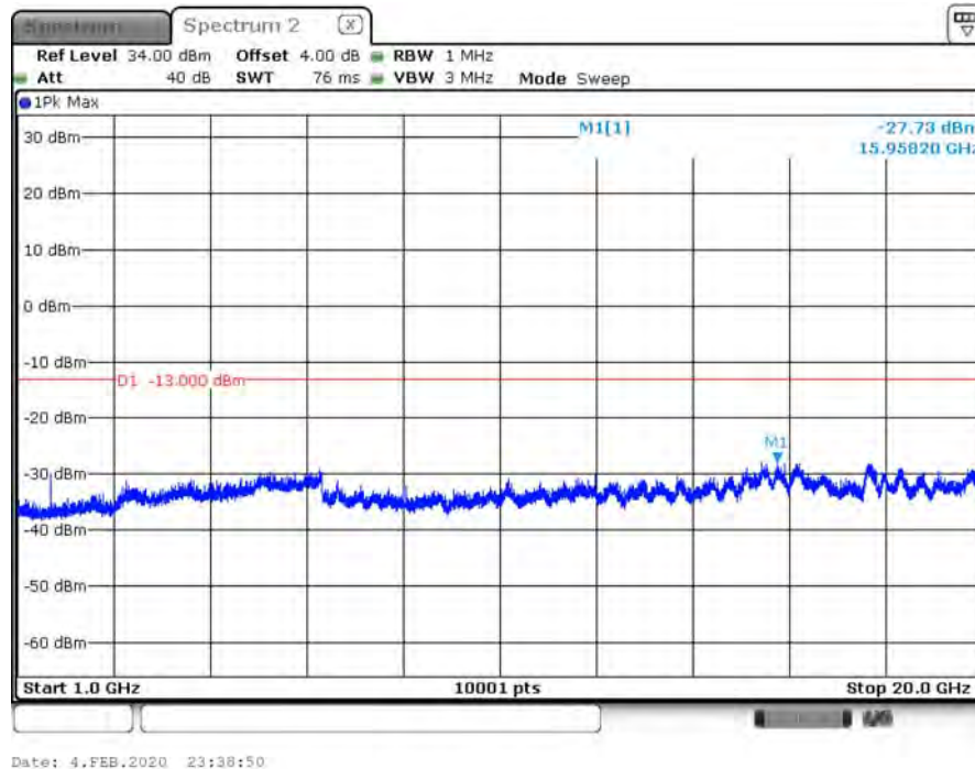
GSM_850_GPRS_824.2_above 1G
