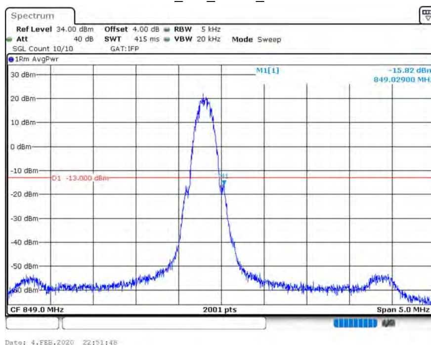
GSM_850_GPRS_848.8
