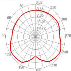
2500.000MHz E2
