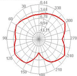
2450.000MHz E2
