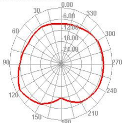
2410.000MHz H
