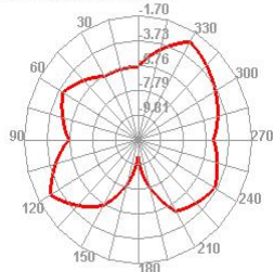
2400.000MHz E2
