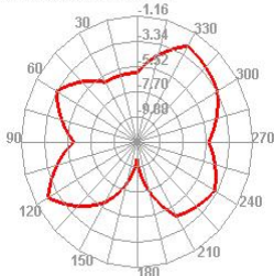
2410.000MHz E2
