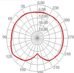
2450.000MHz H
