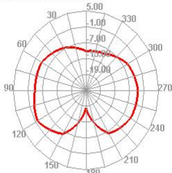
2500.000MHz H
