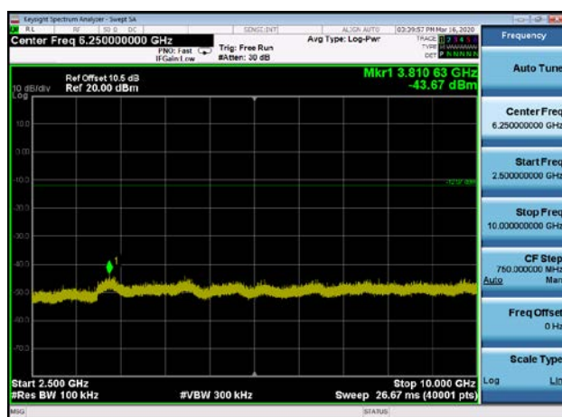
,Plot 4,2500MHz~10000MHz-802.11b ,2437MHz,Ant0
