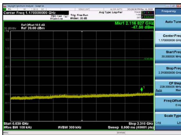
,Plot 3,30MHz~2310MHz-802.11b,2462MHz ,Ant0
