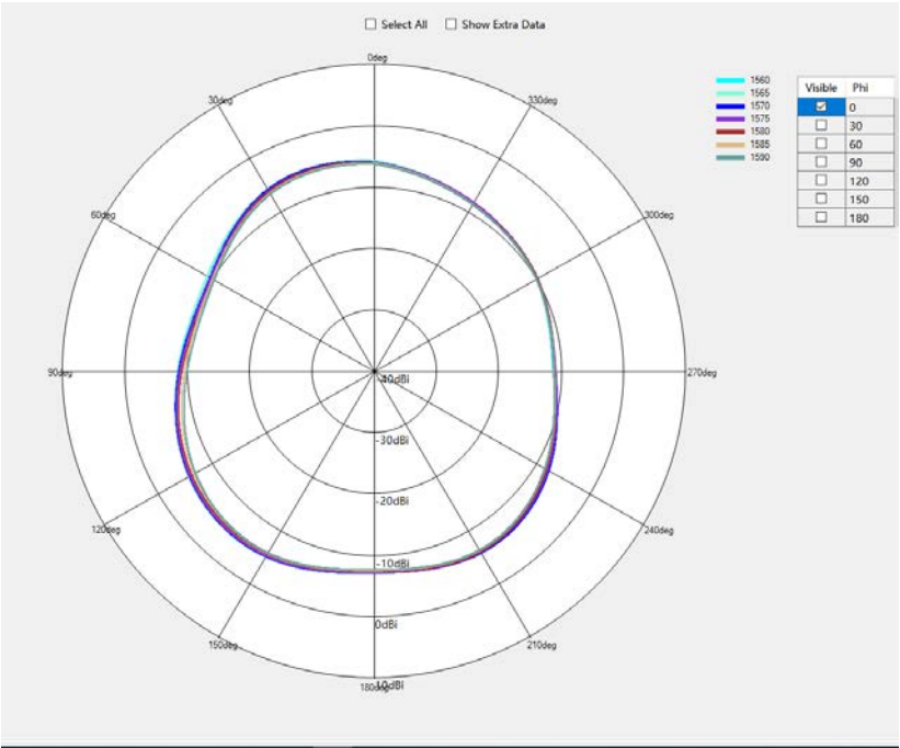
GPS Phi=0deg
