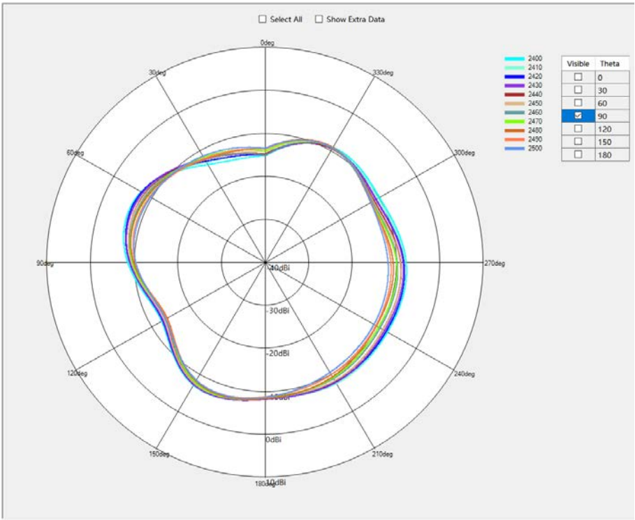
WIFI2.4G Theta=90deg
