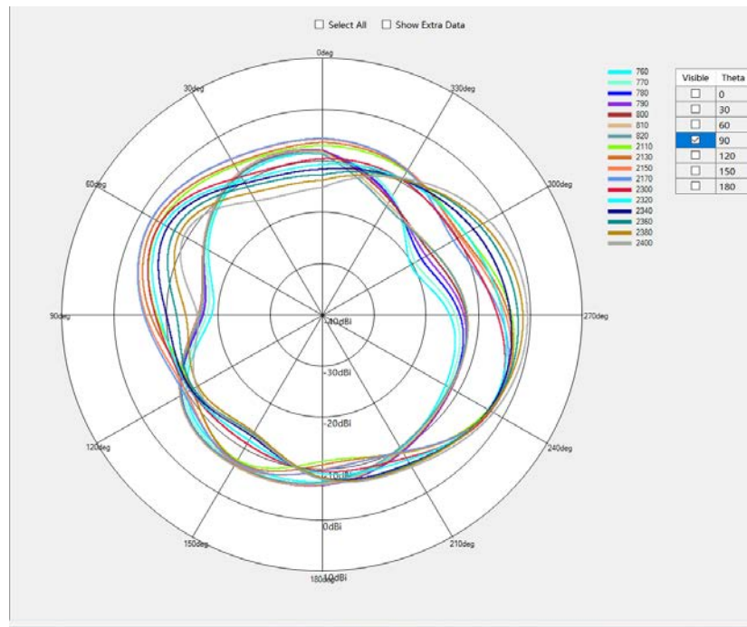
B1/B4/B20/B28/B40/W1/W4 Theta=90deg
