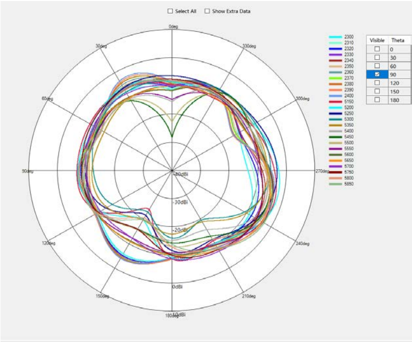
WIFI2.4G/BT/WIFI5G Theta=90deg
