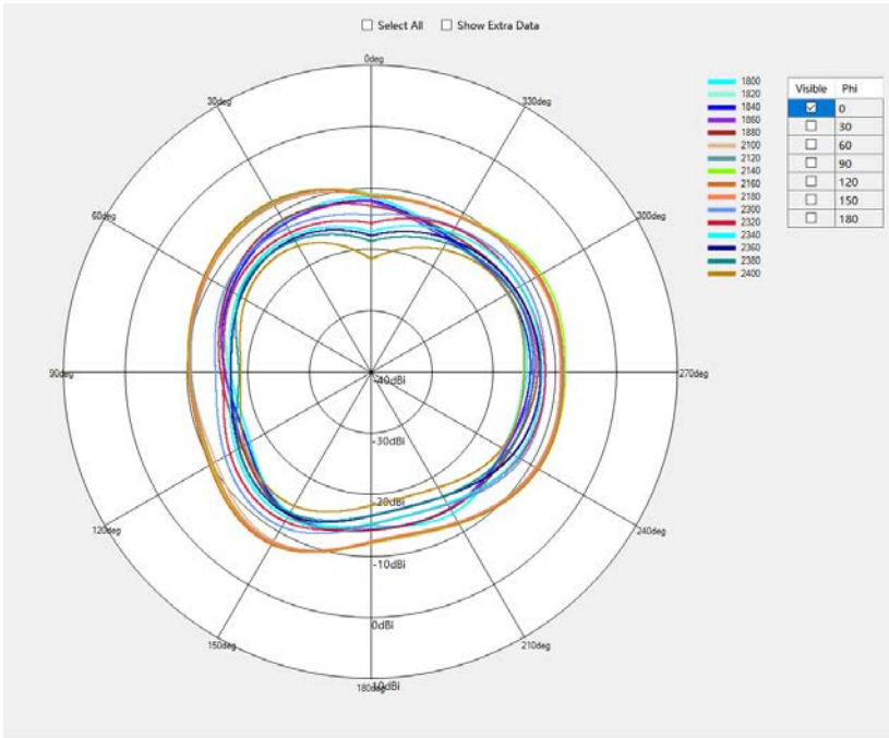
B1/B3/B40 Phi=0deg
