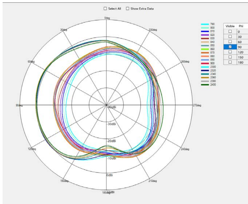
G850/B5/B20/B40/W5 Phi=90deg
