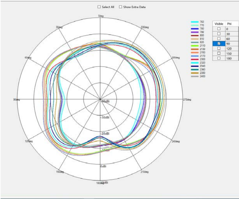
B1/B4/B20/B28/B40/W1/W4 Phi=90deg
