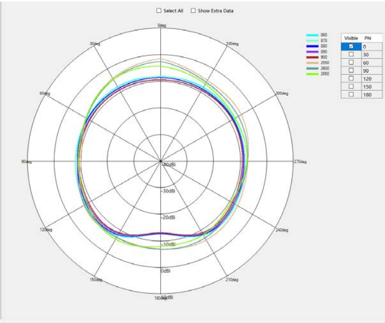
G850/B5/B38/W5 Phi=0deg
