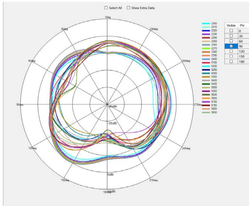
WIFI2.4G/BT/WIFI5G Phi=90deg
