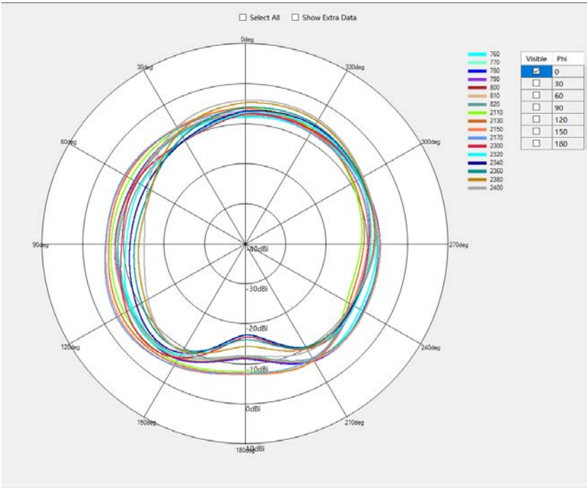
B1/B4/B20/B28/B40/W1/W4 Phi=0deg
