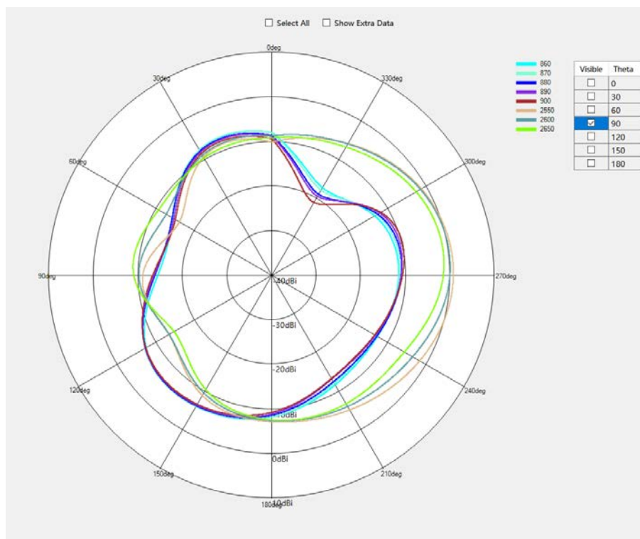
G850/B5/B38/W5 Theta=90deg
