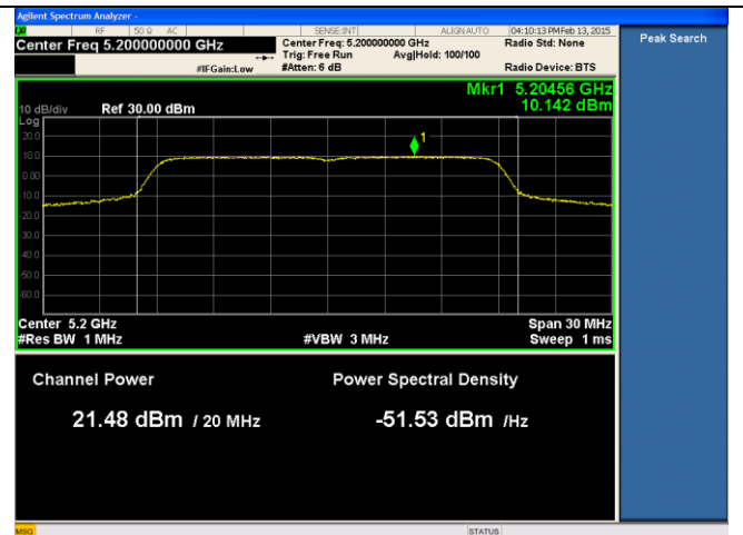
PSD-802.11n HT20-5200M-chain2
