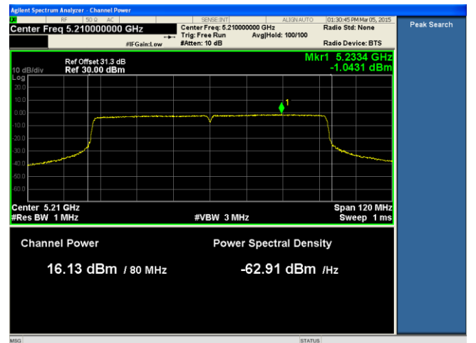
PSD-802.11ac-5210M-chain2
