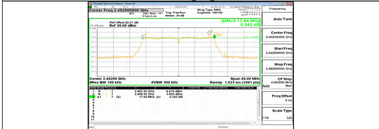
11N20MIMO Ant1 2462
