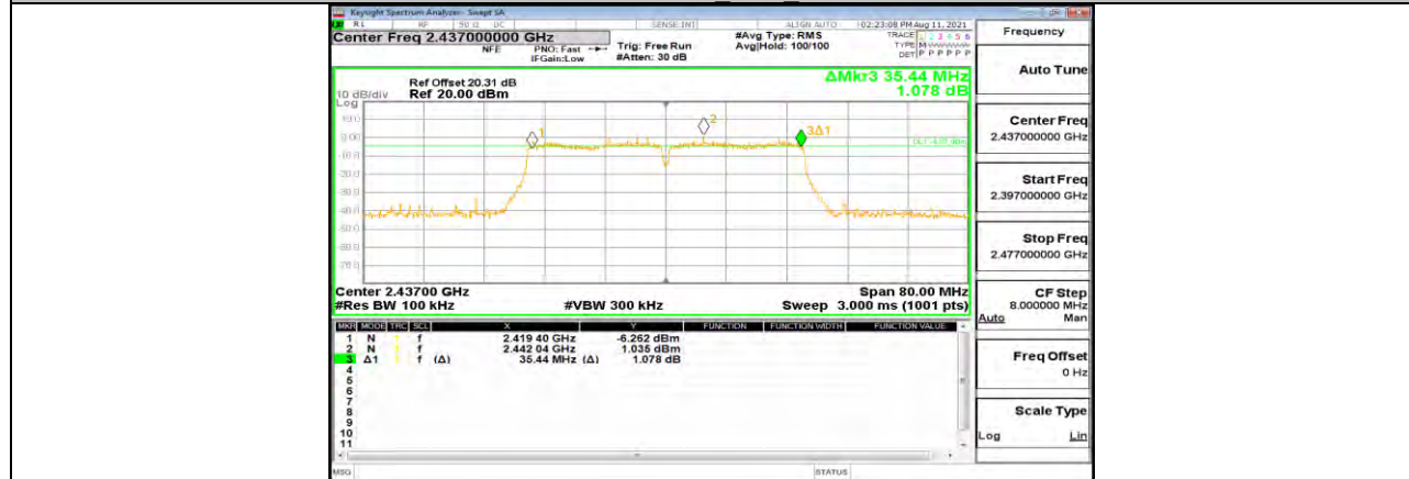
11N40MIMO Ant1 2437
