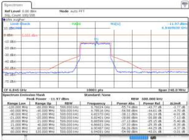
MIMO A-802.11ax/be-40MHz-Ch179-MCS0
