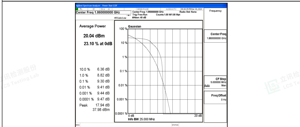
Band2-20MHz-QPSK-18700-1-0-Low-9.30-&lt;=13-PASS
