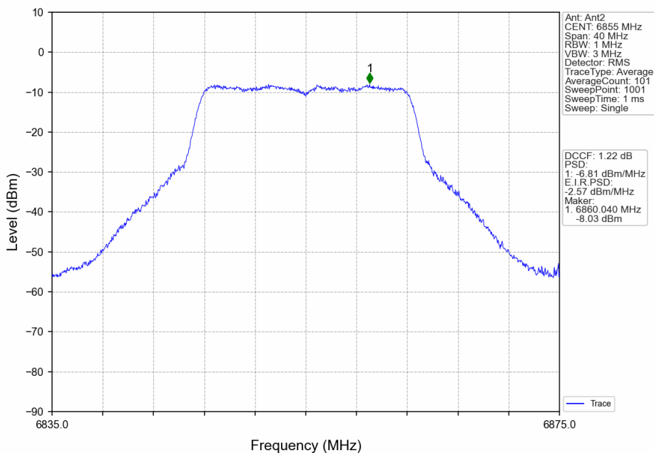
802.11ax(HEW20)_HCH_6855MHz_RU242_Left_Ant2_NTNV
