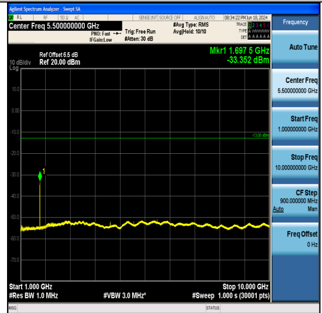
GPRS850-251-5-1000~10000MHz-PASS
