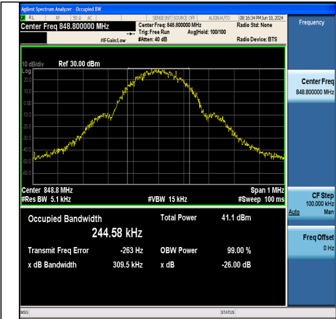
GSM850-251-5-PASS
