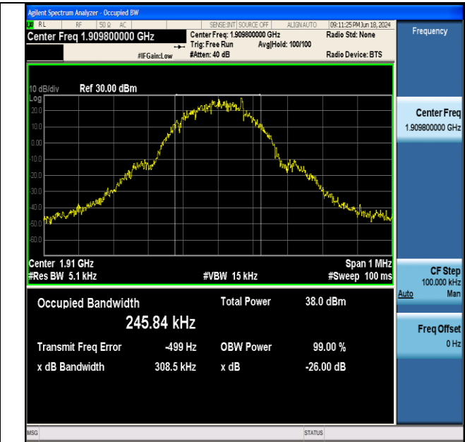
GSM1900-810-0-PASS
