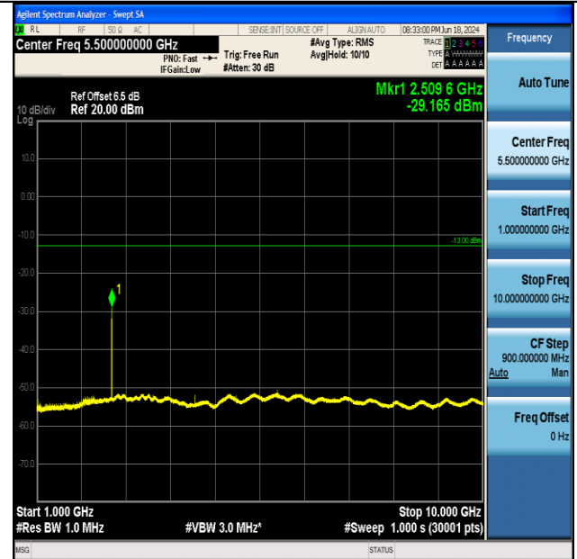
GPRS850-190-5-1000~10000MHz-PASS
