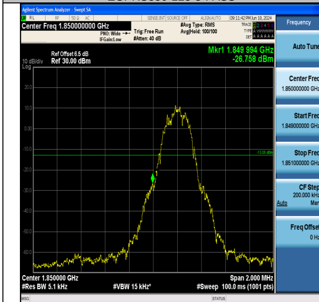
GSM1900-512-0-PASS
