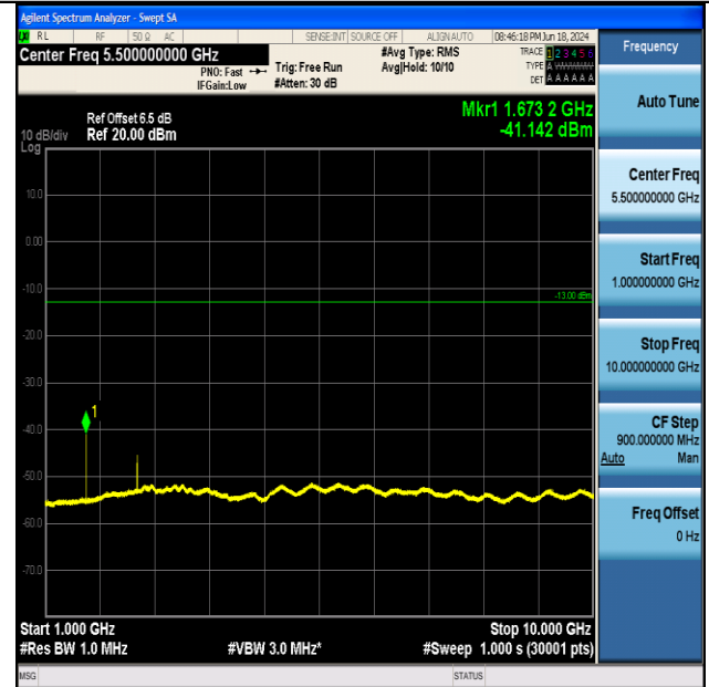
EGPRS850-190-8-1000~10000MHz-PASS
