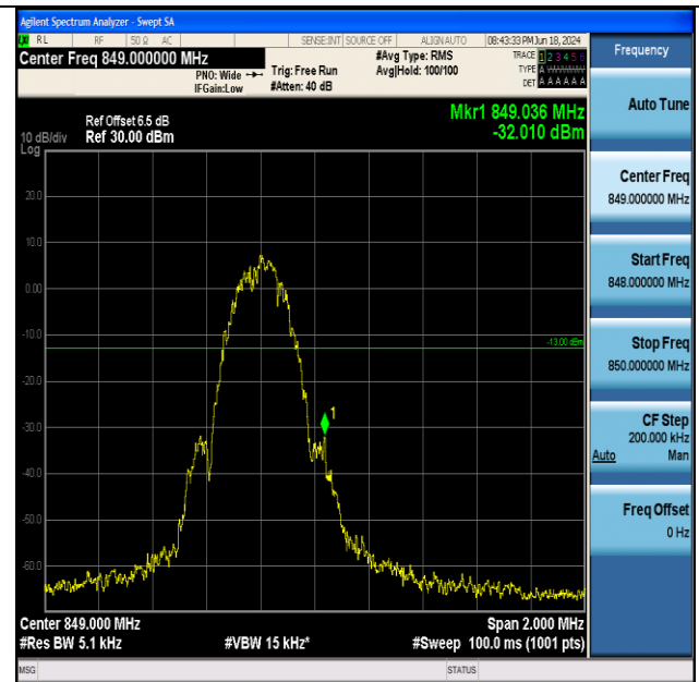
EGPRS850-251-8-PASS
