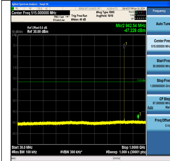
EGPRS850-190-8-30~1000MHz-PASS
