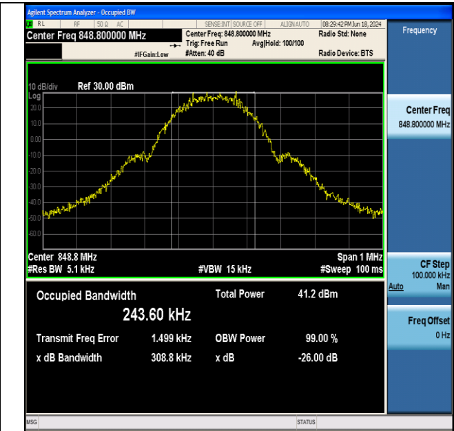
GPRS850-251-5-PASS
