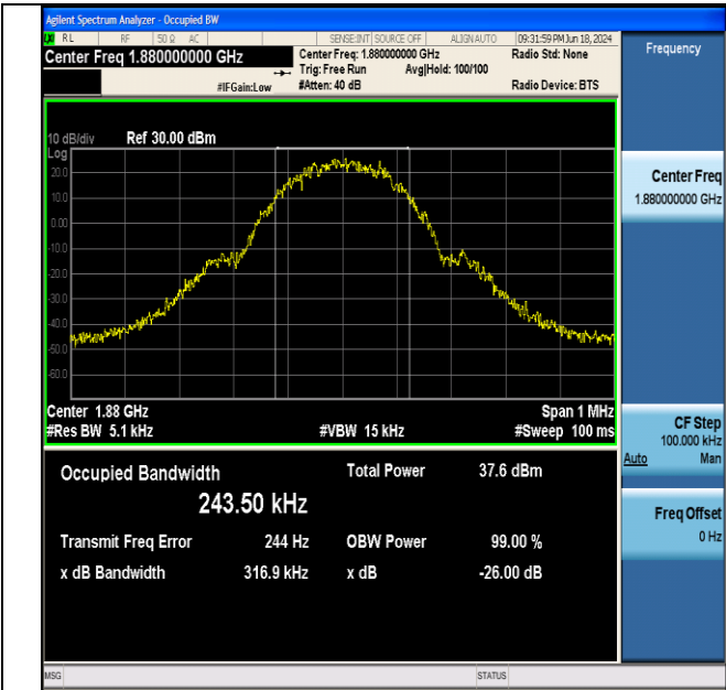
GPRS1900-661-0-PASS
