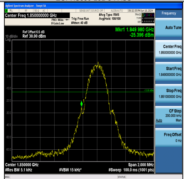
GPRS1900-512-0-PASS
