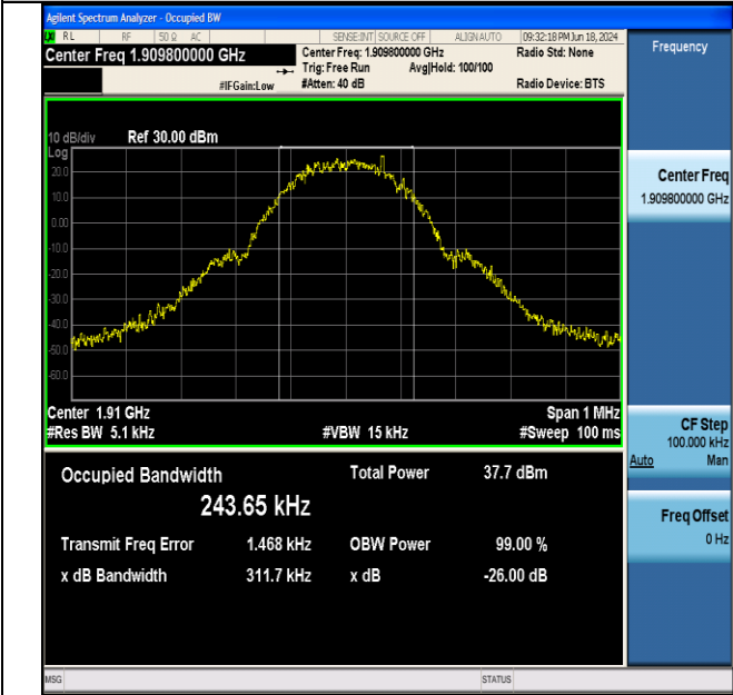
GPRS1900-810-0-PASS
