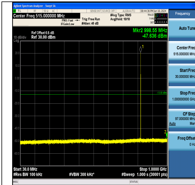
EGPRS850-128-8-30~1000MHz-PASS
