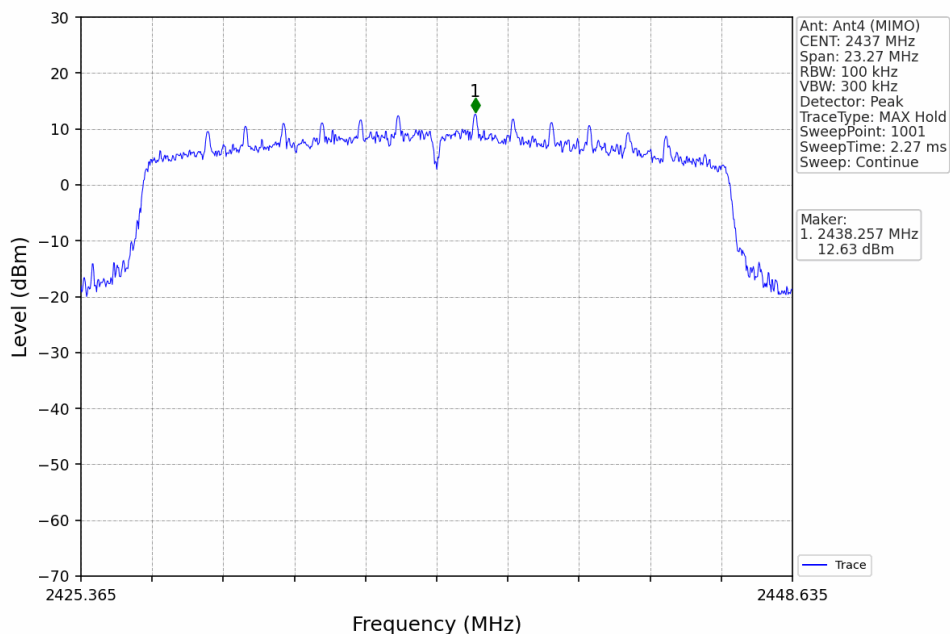
802.11ax(HEW20)_MCH_2437MHz_RU242_Left_Ant4 (MIMO)_NTNV
