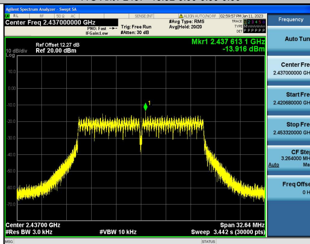
11G-Ant1-2462--14.31-0.00-0.00-0.00
