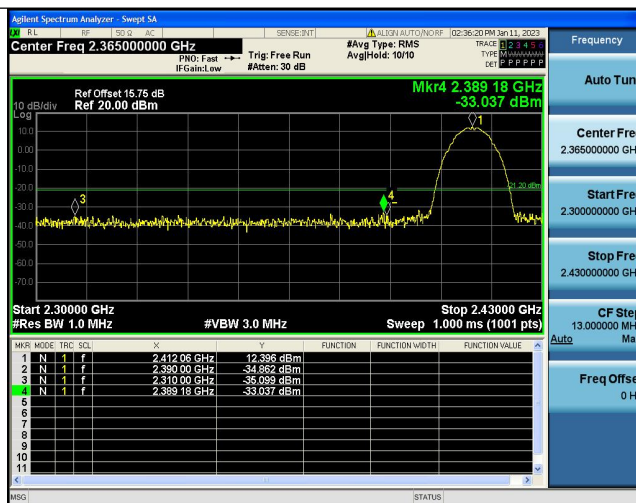
11B-Ant1-Low-2412-AV-2390.000
