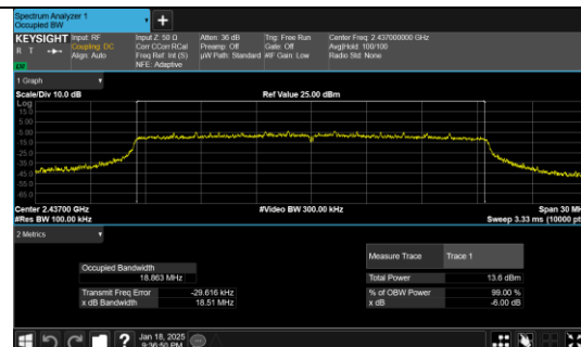
IEEE 802.11ax_Channel 6_20MHz_Antenna 0_RU&Index SU
