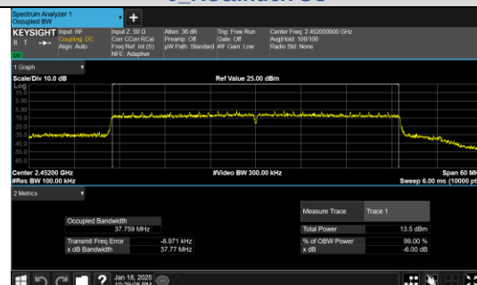
IEEE 802.11ax_Channel 9_40MHz_Antenna 0_RU&Index SU
