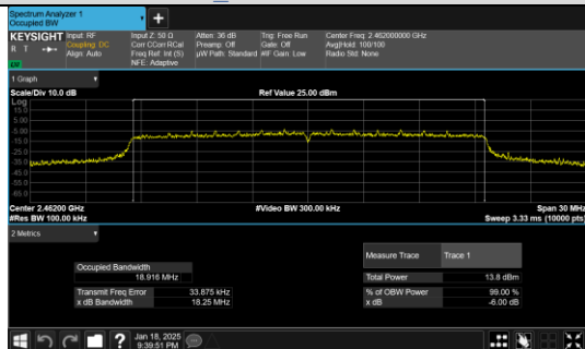
IEEE 802.11ax_Channel 11_20MHz_Antenna 0_RU&Index SU
