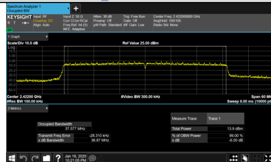
IEEE 802.11ax_Channel 3_40MHz_Antenna 0_RU&Index SU
