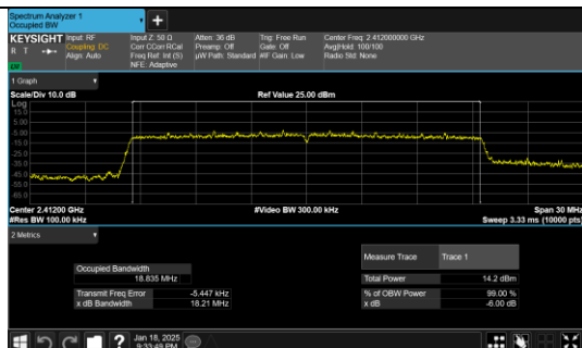
IEEE 802.11ax_Channel 1_20MHz_Antenna 0_RU&Index SU
