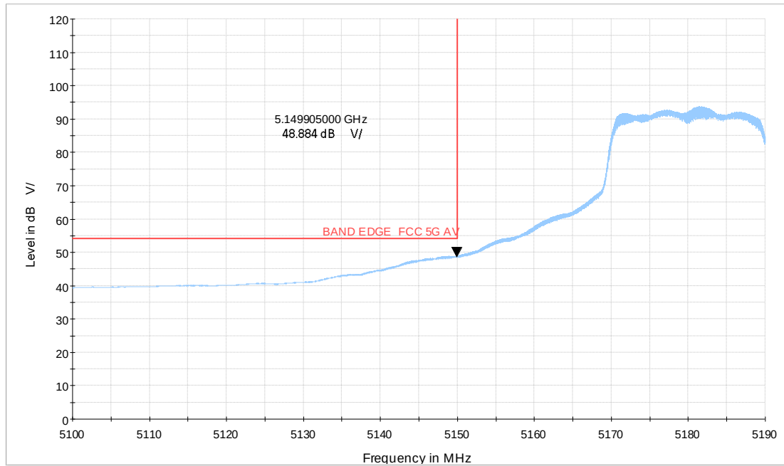
Wi-Fi 5G_ax20 CH36_5.1-5.19GHz_MCS0_MIMO_V_TP22_AV
