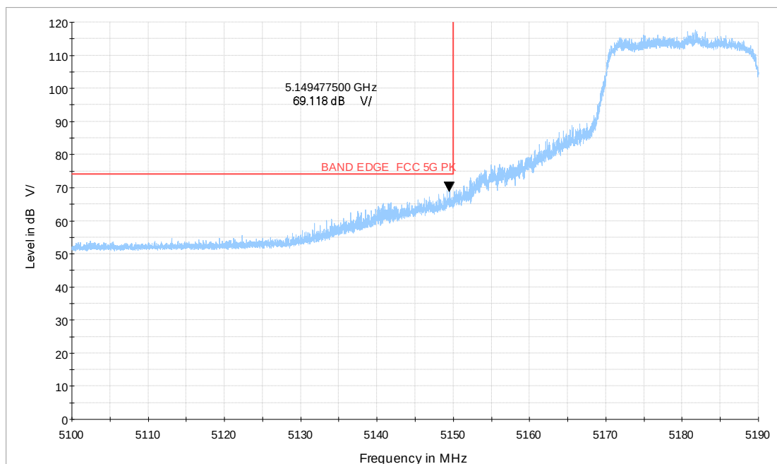
Wi-Fi 5G_ax20 CH36_5.1-5.19GHz_MCS0_MIMO_V_TP22_PK
