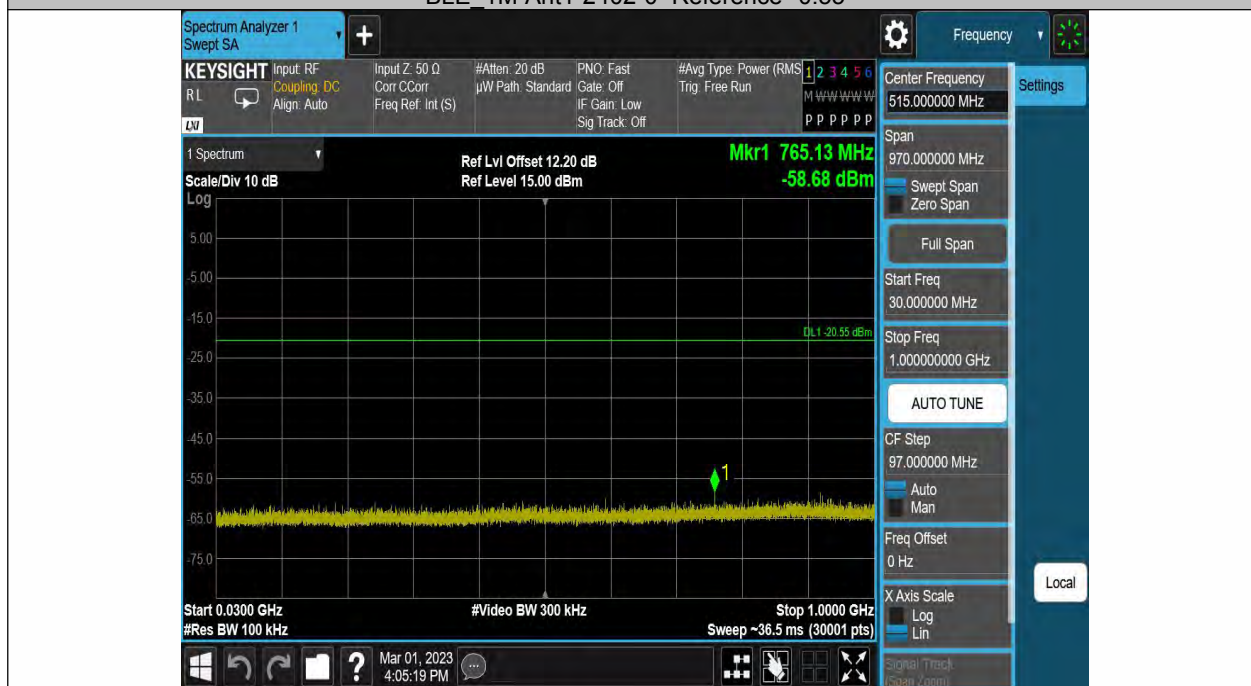
BLE_1M-Ant1-2402-30~1000--0.55
