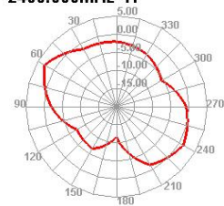
2400.000MHz H
