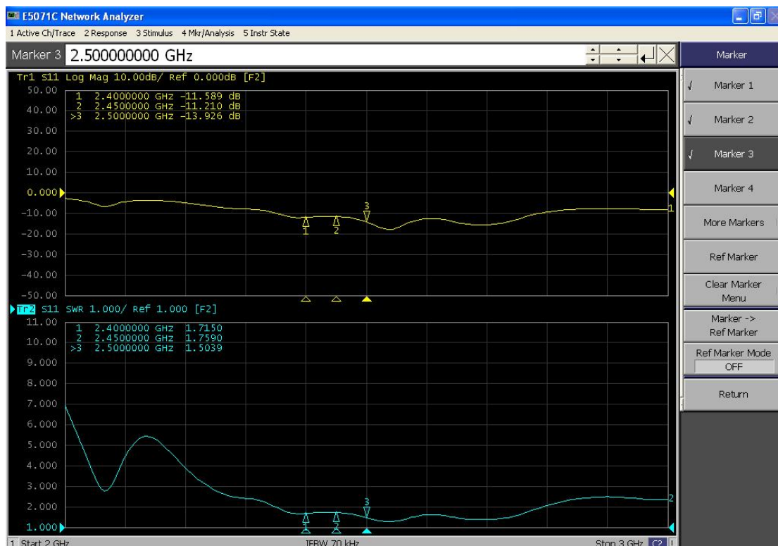
2400.000MHz
