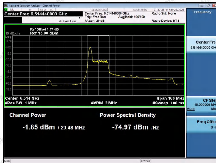
11AX80SISO-Ant1-6545-26Tone-RU0-PASS
