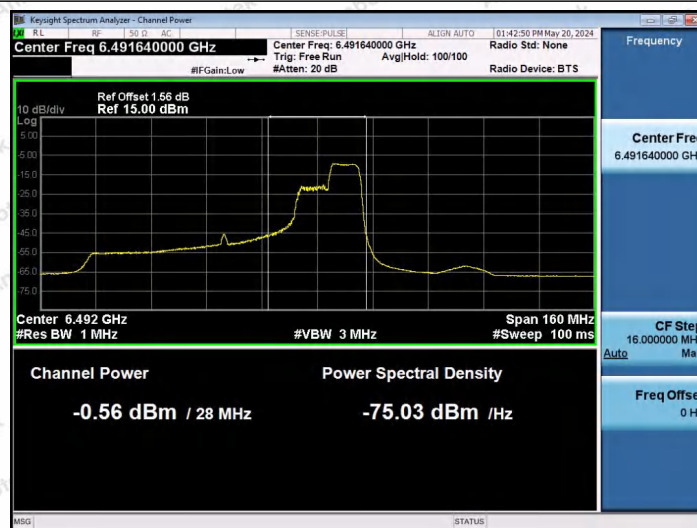
11AX80SISO-Ant1-6465-106Tone-RU60-PASS
