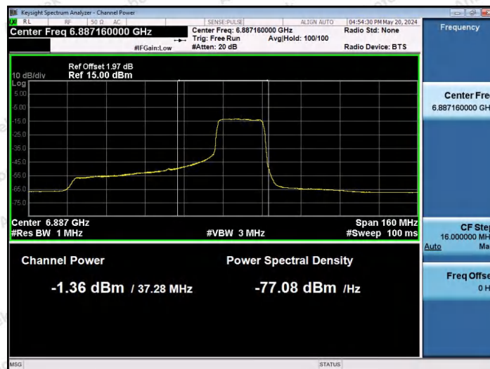
11AX80SISO-Ant1-6865-242Tone-RU64-PASS
