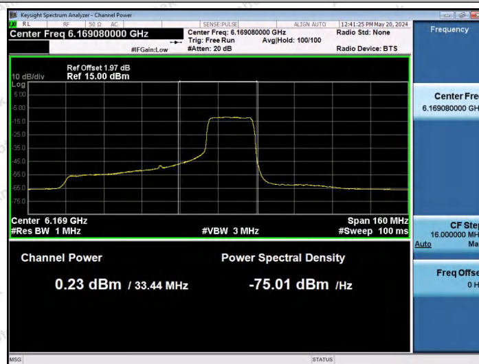
11AX80SISO-Ant1-6145-242Tone-RU64-PASS
