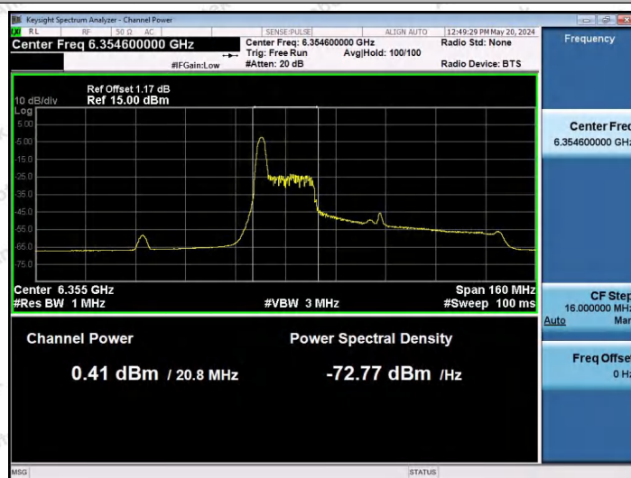
11AX80SISO-Ant1-6385-26Tone-RU0-PASS
