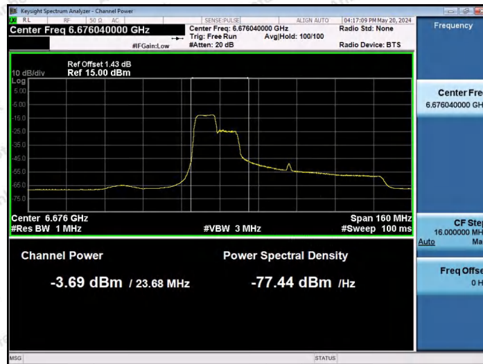
11AX80SISO-Ant1-6705-106Tone-RU53-PASS
