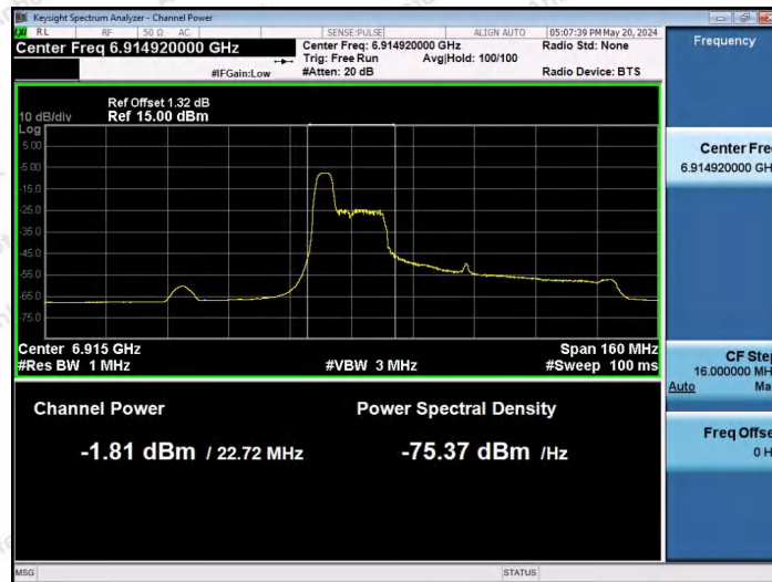
11AX80SISO-Ant1-6945-52Tone-RU37-PASS
