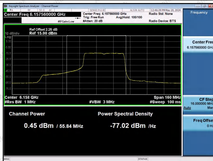
11AX80SISO-Ant1-6145-484Tone-RU66-PASS
