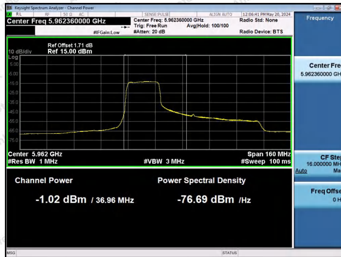
11AX80SISO-Ant1-5985-242Tone-RU61-PASS
