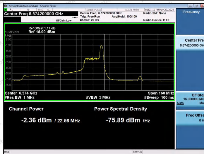
11AX80SISO-Ant1-6545-26Tone-RU36-PASS
