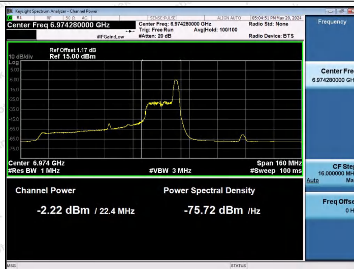
11AX80SISO-Ant1-6945-26Tone-RU36-PASS
