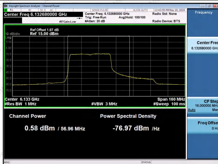
11AX80SISO-Ant1-6145-484Tone-RU65-PASS
