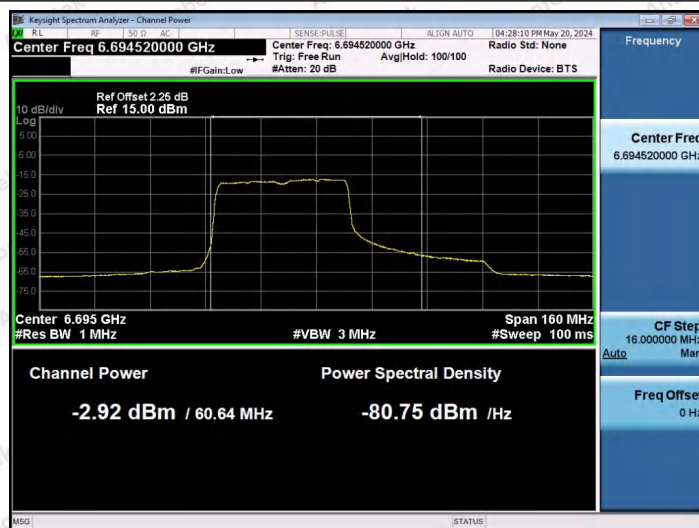
11AX80SISO-Ant1-6705-484Tone-RU65-PASS
