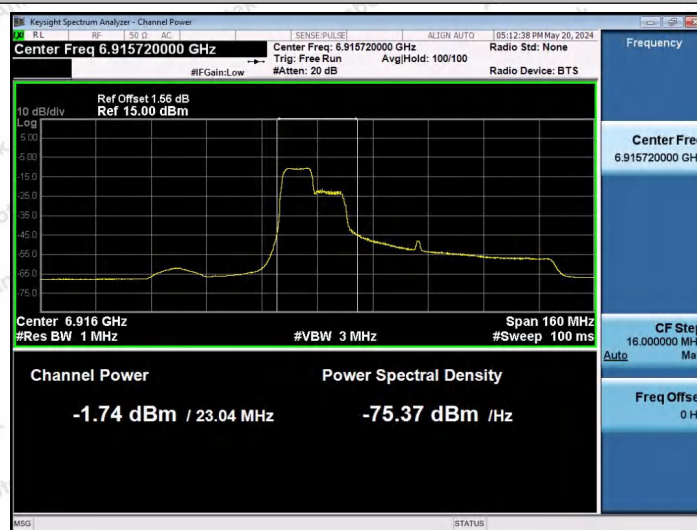
11AX80SISO-Ant1-6945-106Tone-RU53-PASS
