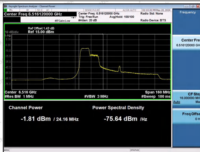
11AX80SISO-Ant1-6545-106Tone-RU53-PASS
