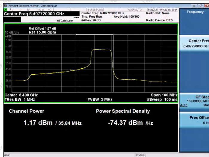
11AX80SISO-Ant1-6385-242Tone-RU64-PASS
