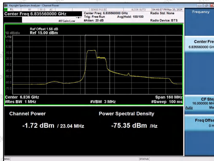
11AX80SISO-Ant1-6865-106Tone-RU53-PASS
