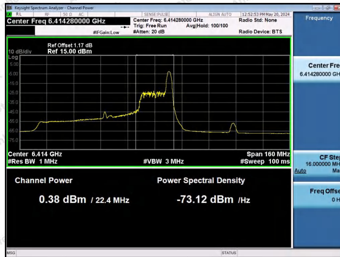
11AX80SISO-Ant1-6385-26Tone-RU36-PASS
