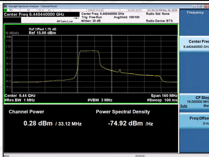
11AX80SISO-Ant1-6465-242Tone-RU61-PASS
