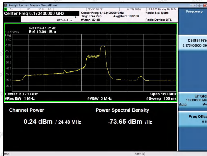
11AX80SISO-Ant1-6145-52Tone-RU52-PASS
