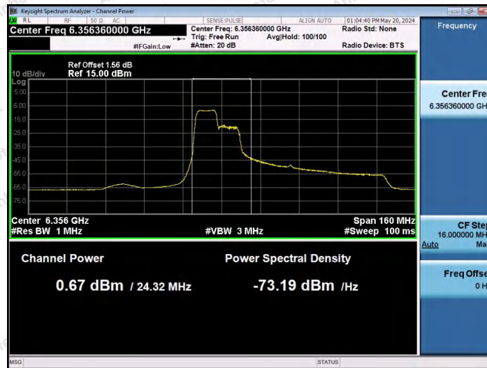
11AX80SISO-Ant1-6385-106Tone-RU53-PASS
