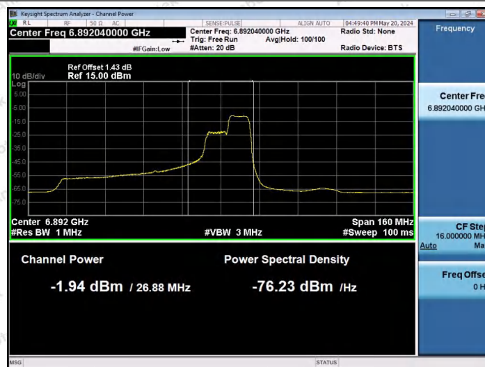
11AX80SISO-Ant1-6865-106Tone-RU60-PASS
