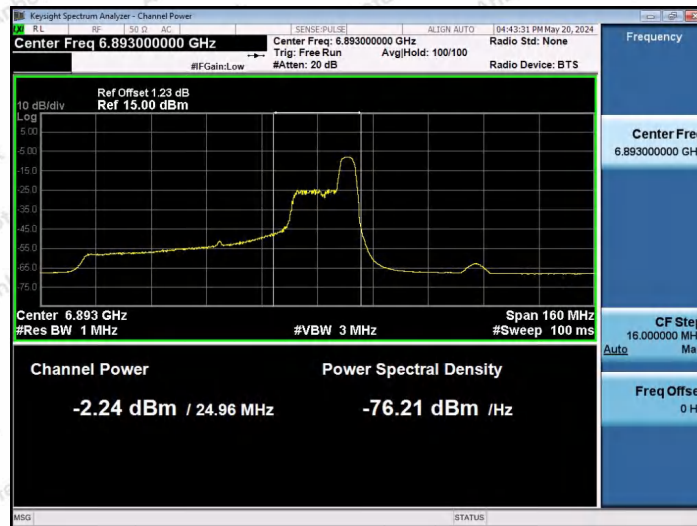
11AX80SISO-Ant1-6865-52Tone-RU52-PASS
