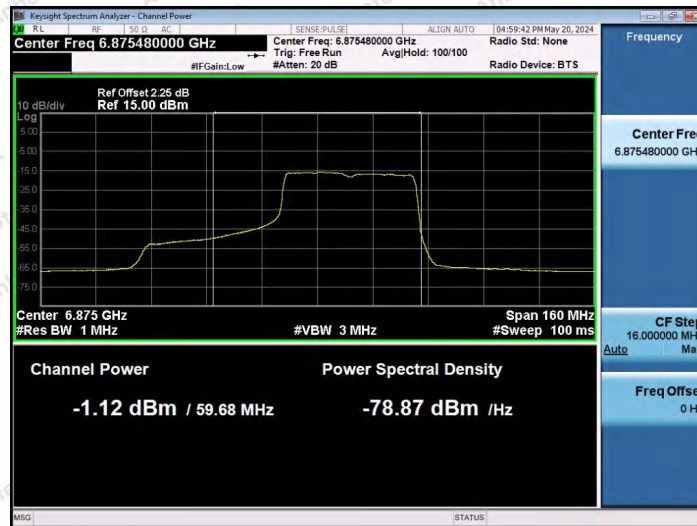
11AX80SISO-Ant1-6865-484Tone-RU66-PASS
