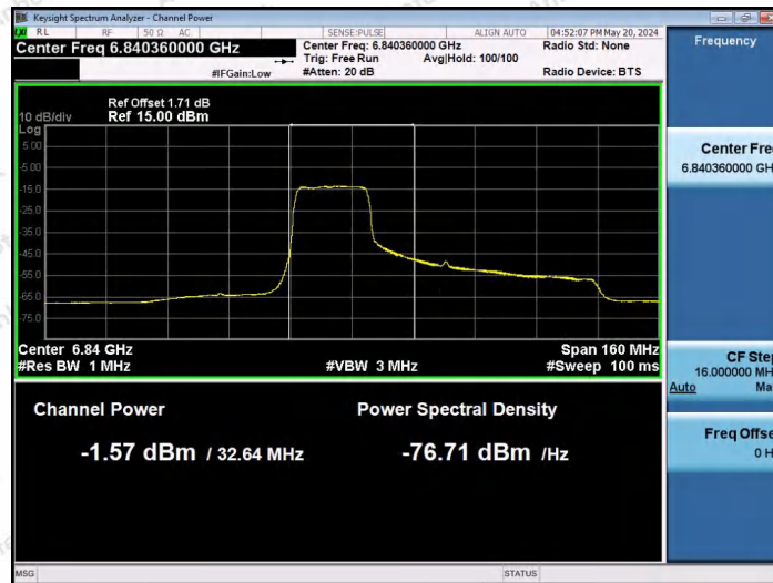
11AX80SISO-Ant1-6865-242Tone-RU61-PASS
