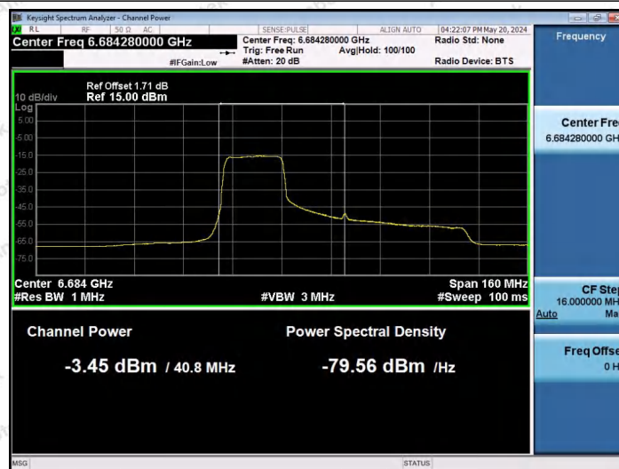
11AX80SISO-Ant1-6705-242Tone-RU61-PASS
