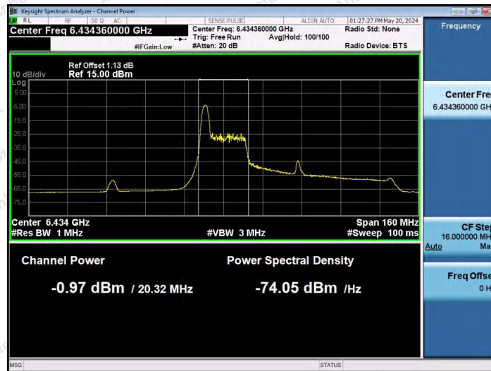
11AX80SISO-Ant1-6465-26Tone-RU0-PASS
