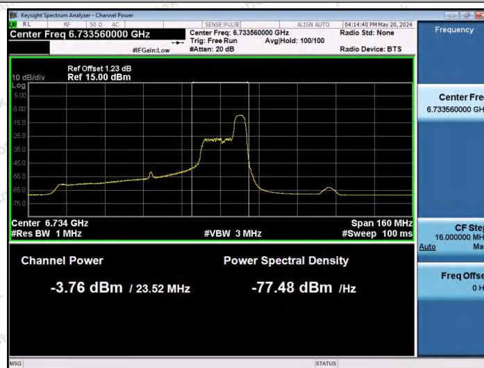
11AX80SISO-Ant1-6705-52Tone-RU52-PASS
