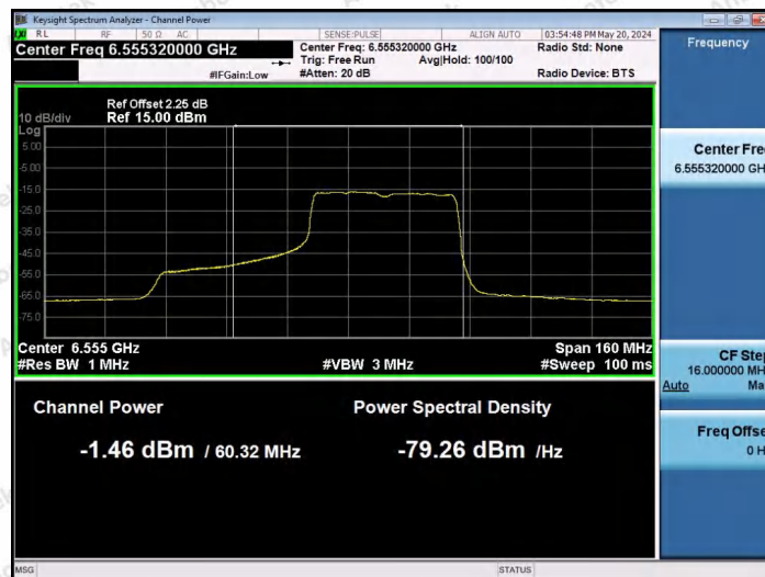
11AX80SISO-Ant1-6545-484Tone-RU66-PASS
