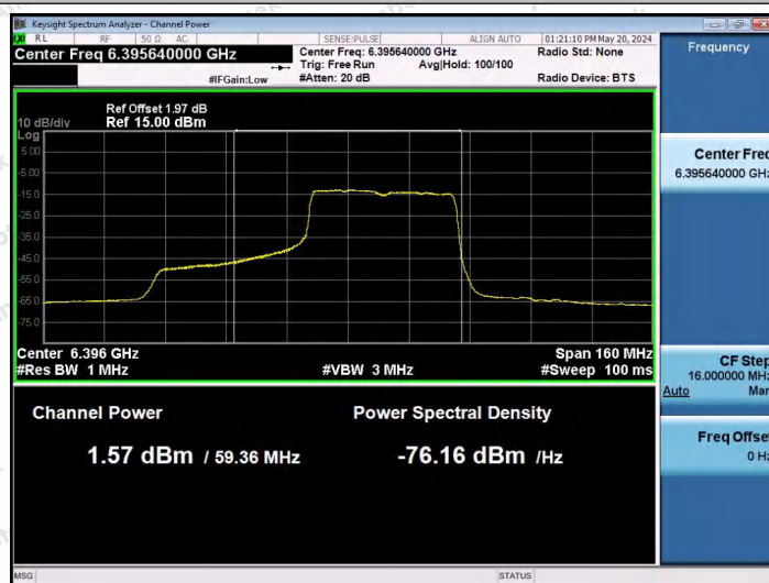
11AX80SISO-Ant1-6385-484Tone-RU66-PASS
