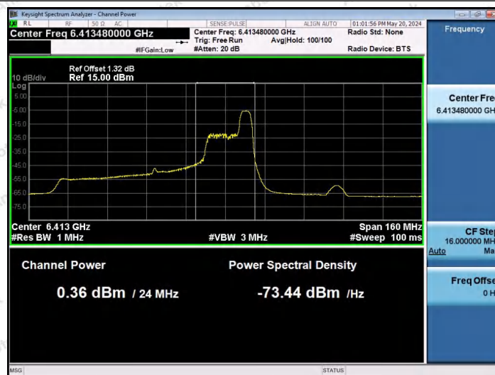
11AX80SISO-Ant1-6385-52Tone-RU52-PASS
