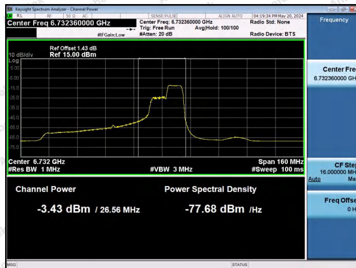
11AX80SISO-Ant1-6705-106Tone-RU60-PASS
