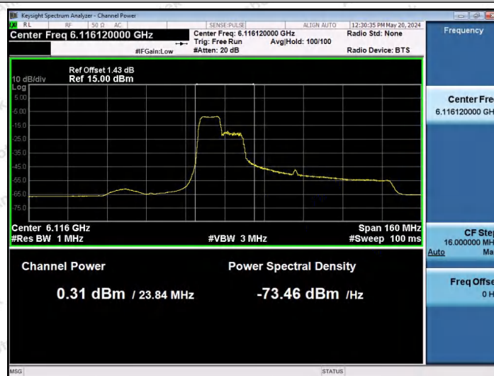
11AX80SISO-Ant1-6145-106Tone-RU53-PASS
