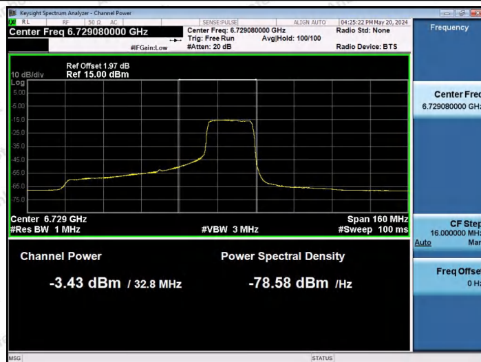
11AX80SISO-Ant1-6705-242Tone-RU64-PASS
