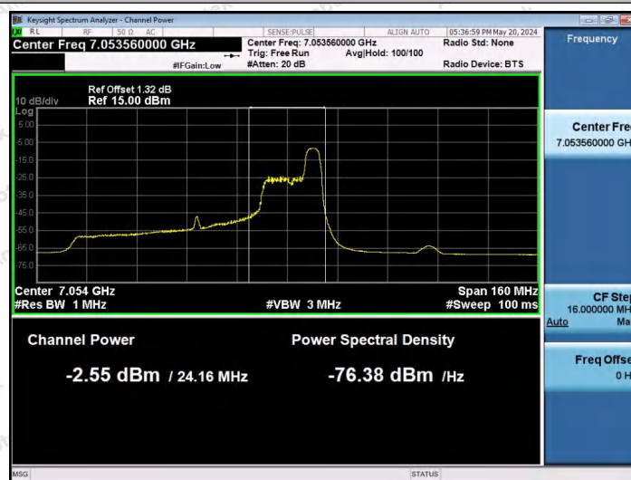
11AX80SISO-Ant1-7025-52Tone-RU52-PASS
