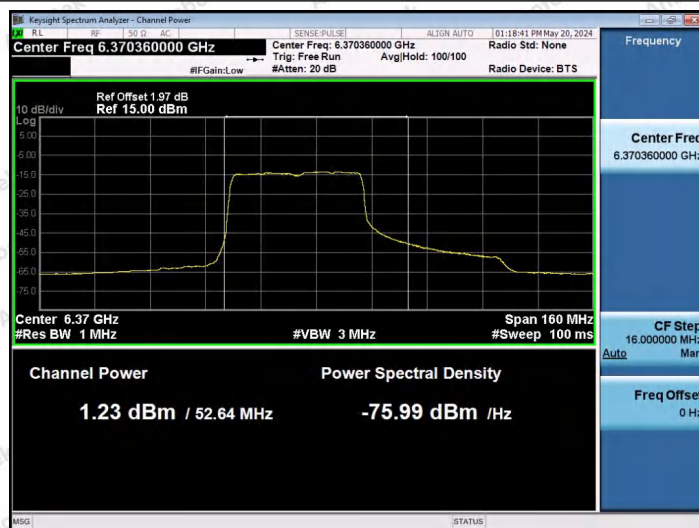
11AX80SISO-Ant1-6385-484Tone-RU65-PASS
