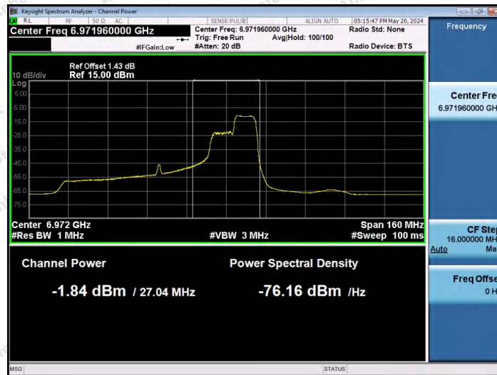
11AX80SISO-Ant1-6945-106Tone-RU60-PASS
