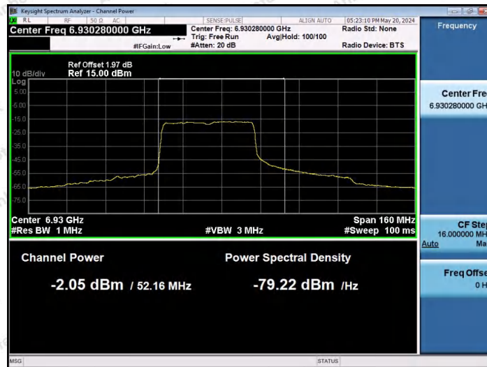
11AX80SISO-Ant1-6945-484Tone-RU65-PASS
