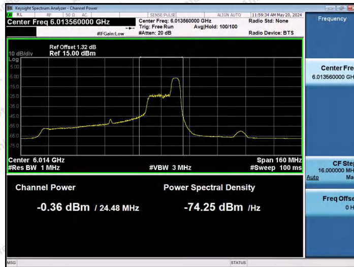
11AX80SISO-Ant1-5985-52Tone-RU52-PASS
