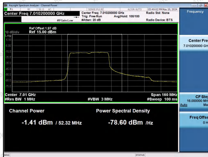
11AX80SISO-Ant1-7025-484Tone-RU65-PASS
