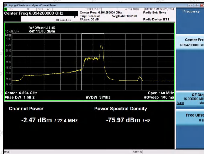
11AX80SISO-Ant1-6865-26Tone-RU36-PASS
