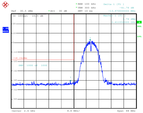
802.11b_2412MHz_Chain 0
