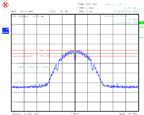
802.11b_2462MHz_Chain 0
