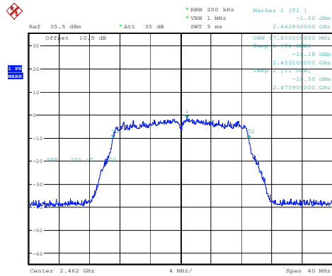
802.11n20_2462MHz_Chain 0
