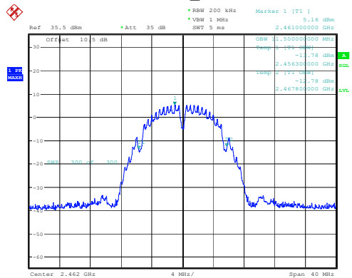
802.11b_2462MHz
