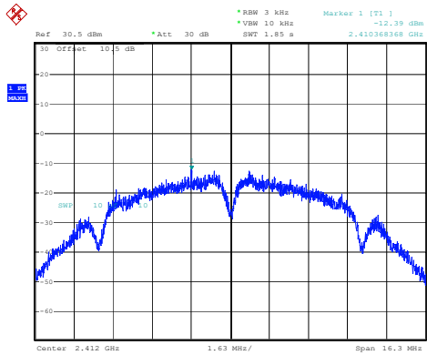
802.11b_2412MHz_Chain 1
