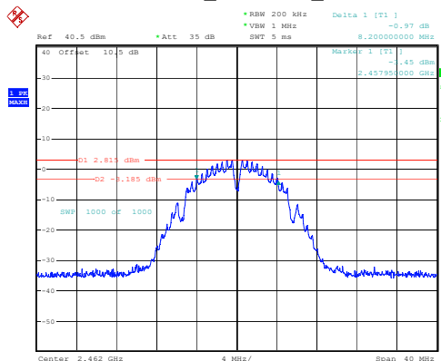
802.11b_2462MHz_Chain 1
