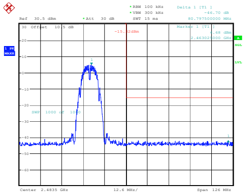
802.11b_2462MHz
