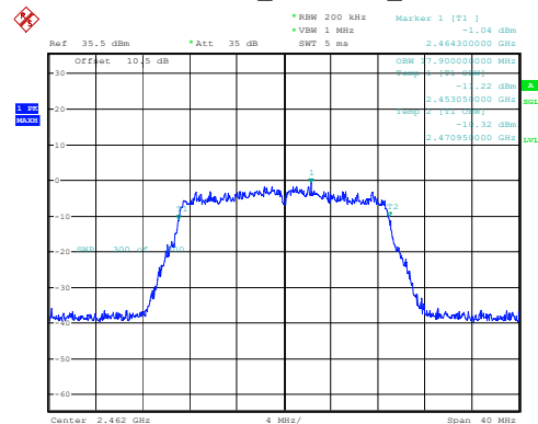
802.11n20_2462MHz_Chain 1
