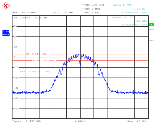
802.11b_2437MHz_Chain 1
