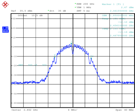
802.11b_2462MHz_Chain 1
