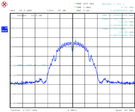
802.11b_2437MHz
