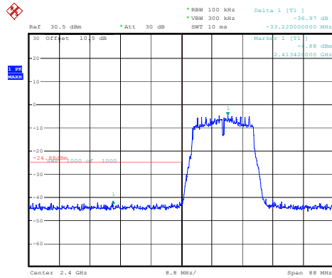
802.11n20_2412MHz_Chain 0
