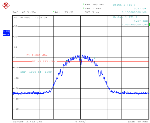
802.11b_2412MHz_Chain 1
