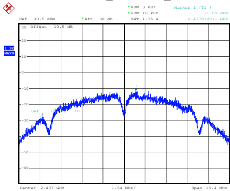
802.11b_2437MHz_Chain 0
