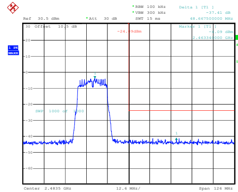
802.11n20_2462MHz_Chain 0
