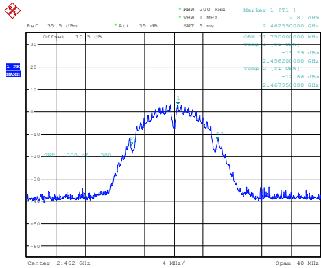
802.11b_2462MHz_Chain 0
