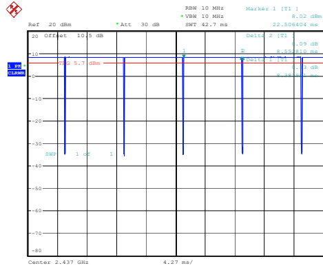
802.11b_2437MHz_Chain 0
