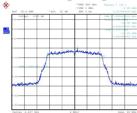
802.11n20_2437MHz_Chain 1
