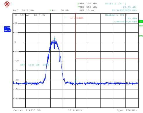
802.11b_2462MHz_Chain 1
