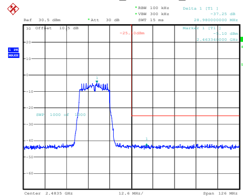
802.11n20_2462MHz_Chain 1
