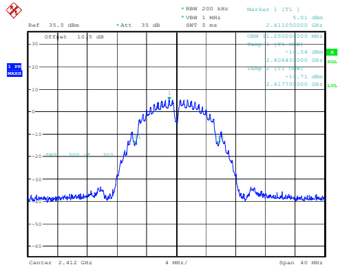
802.11b_2412MHz
