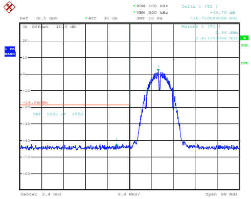
802.11b_2412MHz_Chain 1
