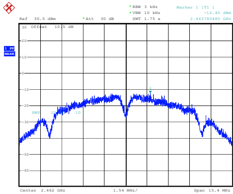
802.11b_2462MHz_Chain 1
