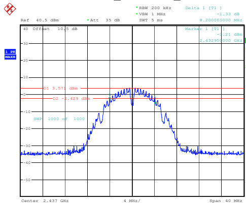
802.11b_2437MHz_Chain 0
