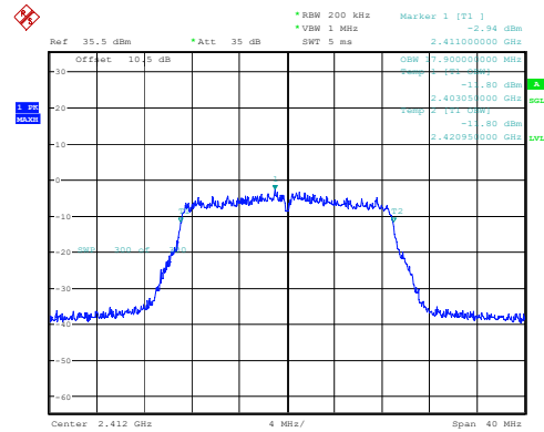
802.11n20_2412MHz_Chain 1
