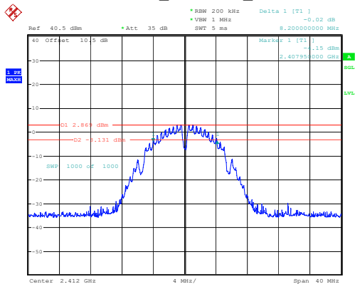
802.11b_2412MHz_Chain 0
