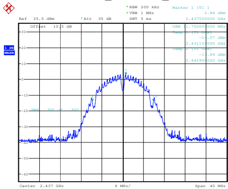
802.11b_2437MHz_Chain 0
