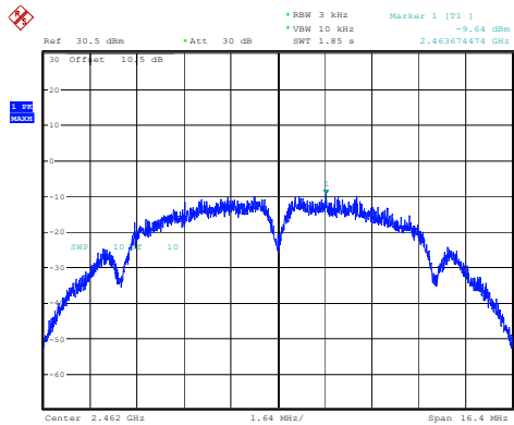
802.11b_2462MHz
