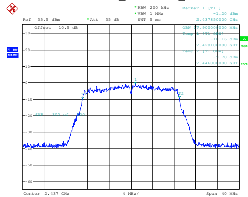
802.11n20_2437MHz_Chain 0
