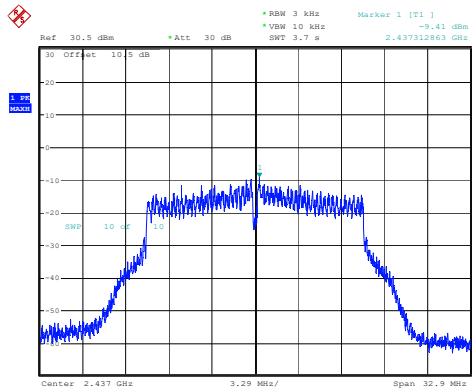
802.11g_2437MHz
