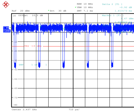
802.11n20_2437MHz_Chain 0
