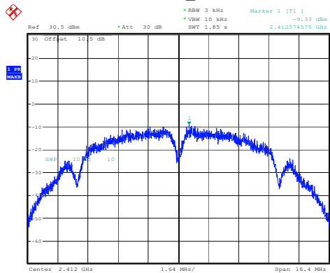
802.11b_2412MHz
