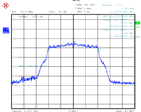
802.11g_2437MHz
