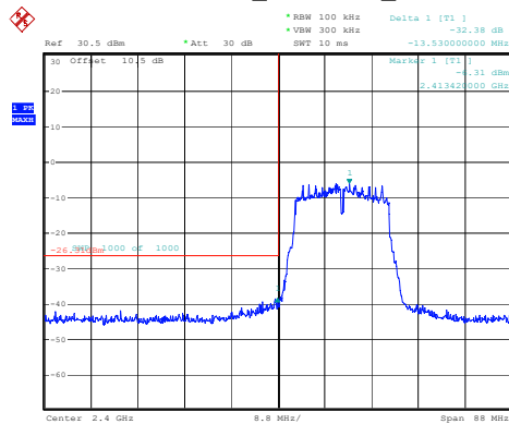
802.11n20_2412MHz_Chain 1
