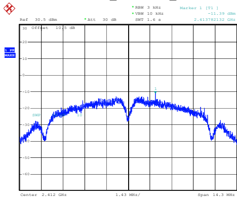
802.11b_2412MHz_Chain 0
