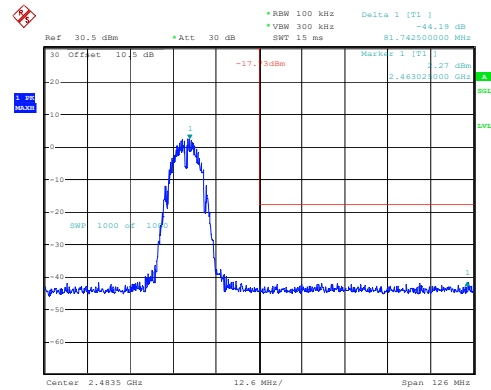
802.11b_2462MHz_Chain 0
