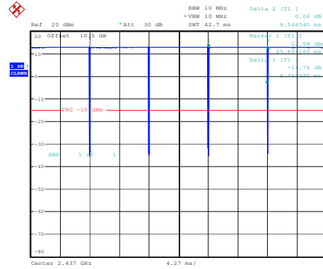
802.11b_2437MHz_Chain 1
