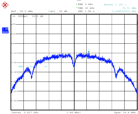
802.11b_2437MHz
