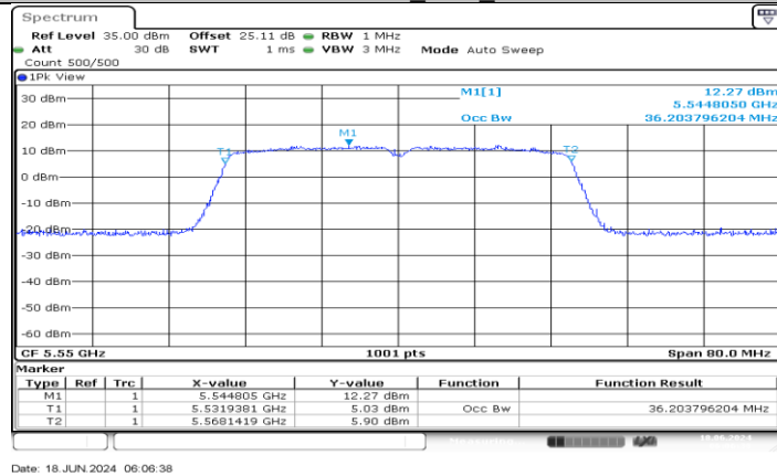
11AC40MIMO_Ant1_5550
