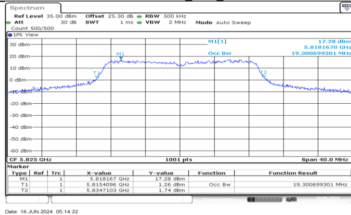
11AC20MIMO_Ant4_5825
