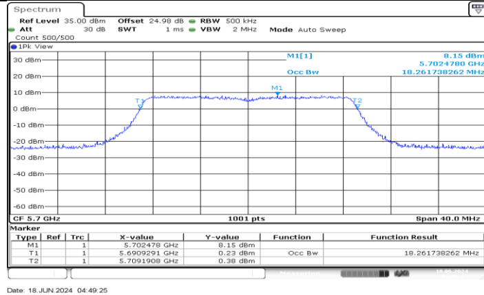
11AC20MIMO_Ant1_5700
