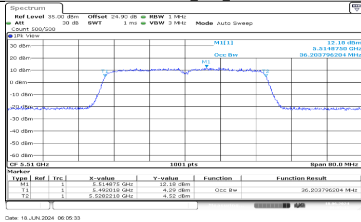
11AC40MIMO_Ant4_5510
