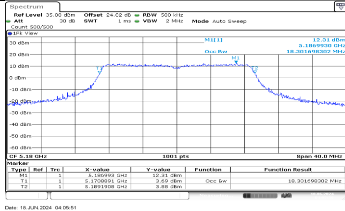
11AC20MIMO_Ant3_5180
