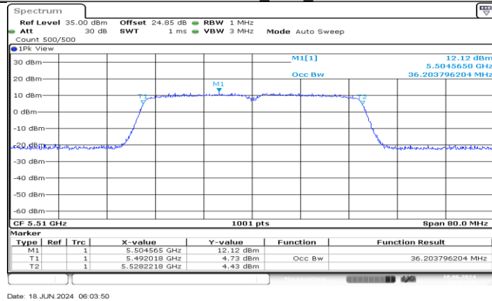
11AC40MIMO_Ant2_5510
