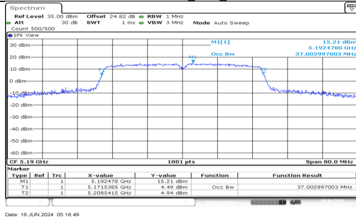
11AC40MIMO_Ant3_5190
