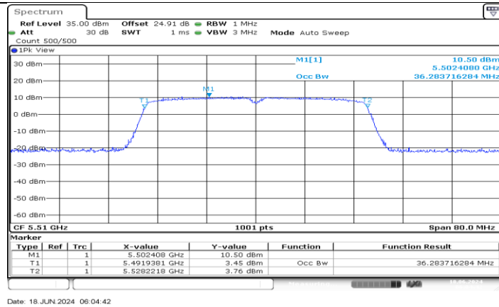
11AC40MIMO_Ant3_5510
