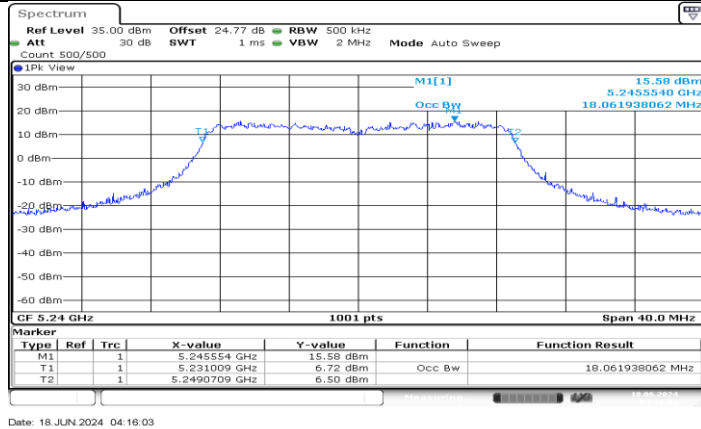
11AC20MIMO_Ant4_5240
