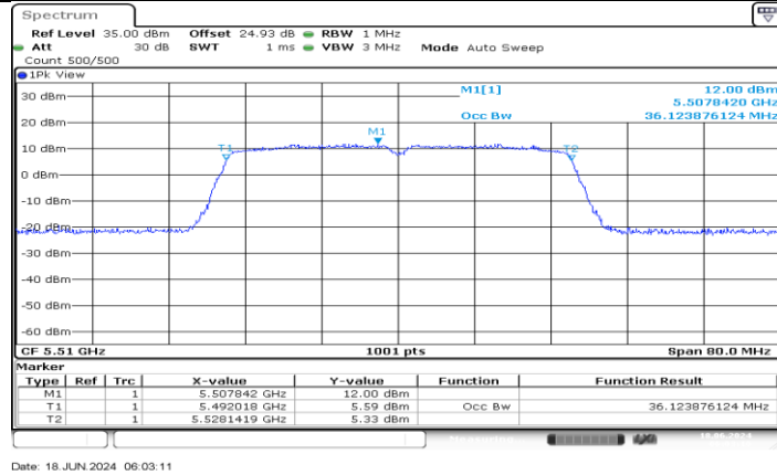
11AC40MIMO_Ant1_5510
