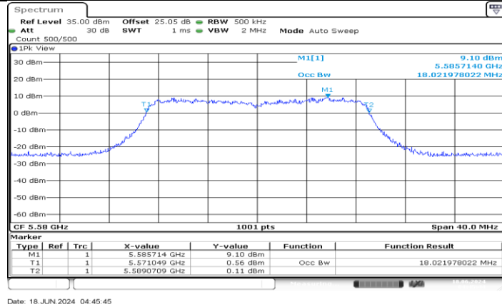
11AC20MIMO_Ant4_5580
