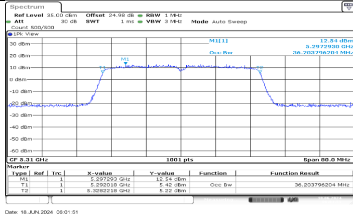
11AC40MIMO_Ant4_5310
