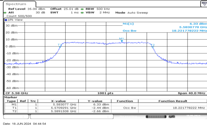
11AC20MIMO_Ant3_5580
