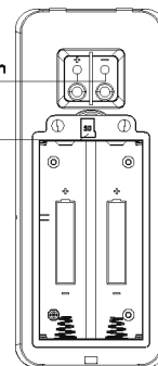
Interface d'alimentation Fente pour carte SD
