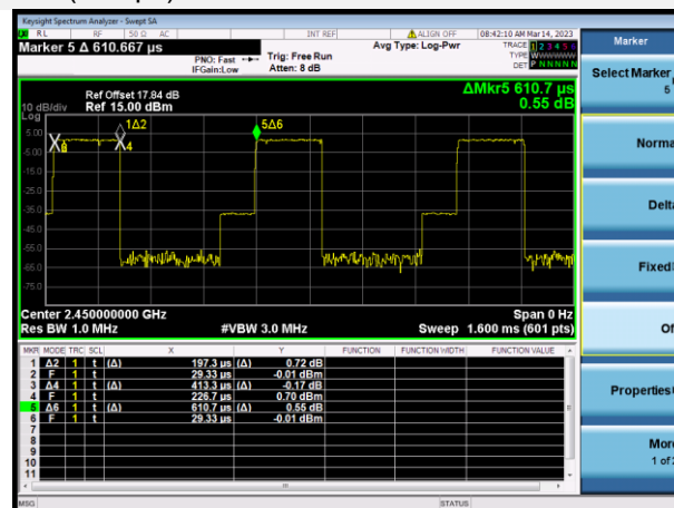
FSK(2Mbps)
