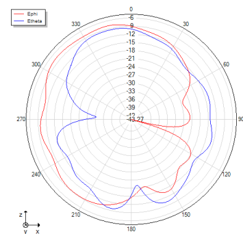
2402MHz
