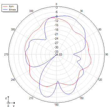
2440MHz
