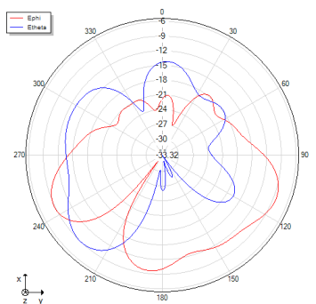
2480MHz
