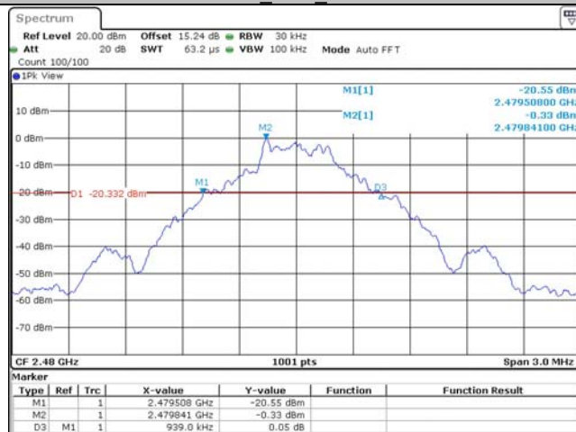
DH1_Ant1_2480
