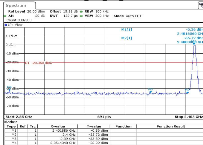
DH1_Ant1_Low_2402
