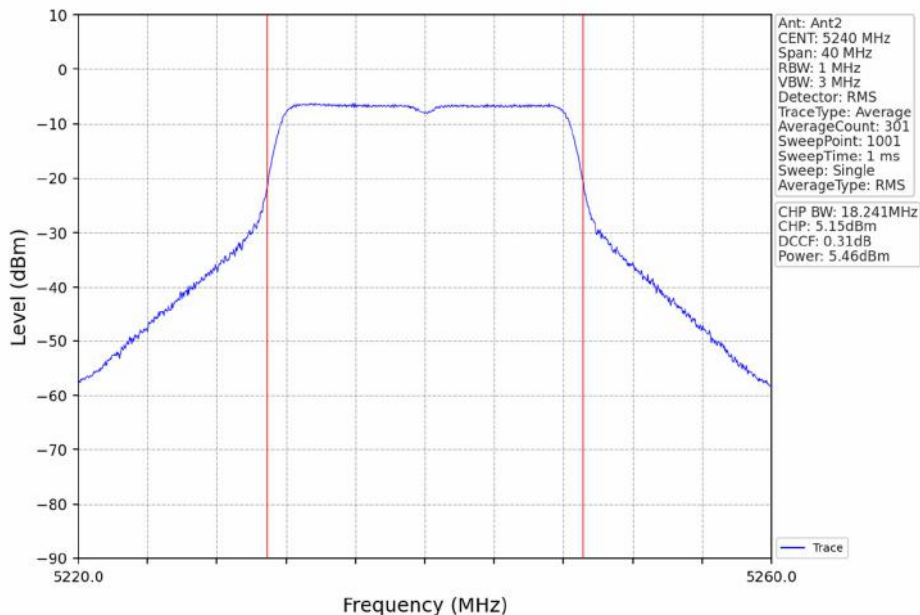
802.11a_HCH_5240MHz_Ant2_NTNV
