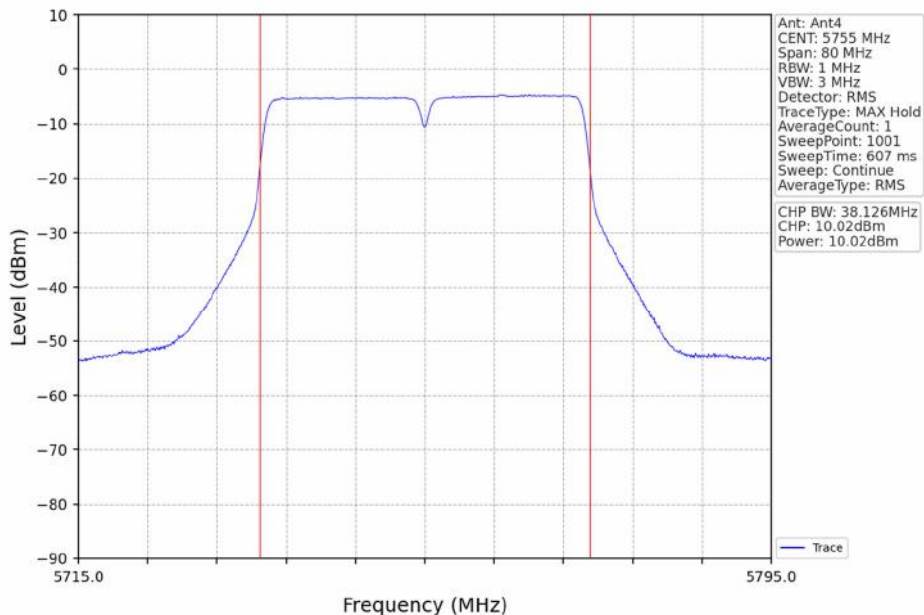
802.11ac(VHT40)_LCH_5755MHz_Ant4_NTNV
