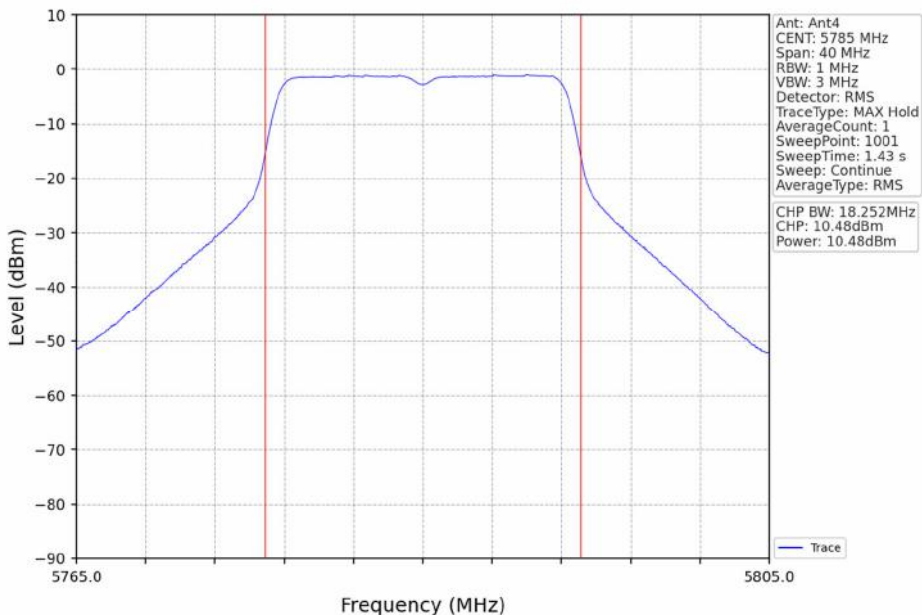
802.11a_MCH_5785MHz_Ant4_NTNV
