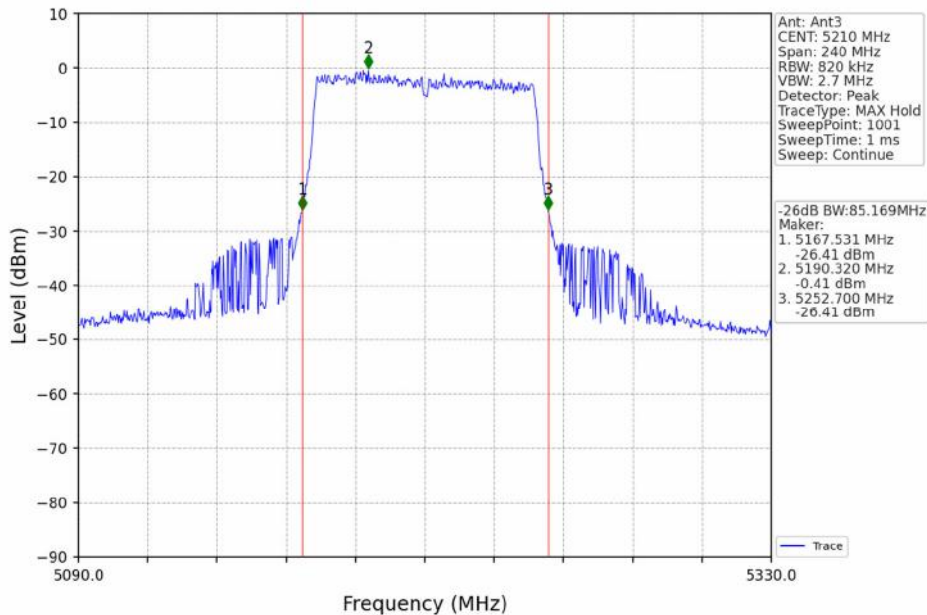
802.11ac(VHT80)_MCH_5210MHz_Ant3_NTNV
