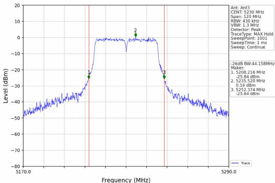
802.11n(HT40)_HCH_5230MHz_Ant3_NTNV
