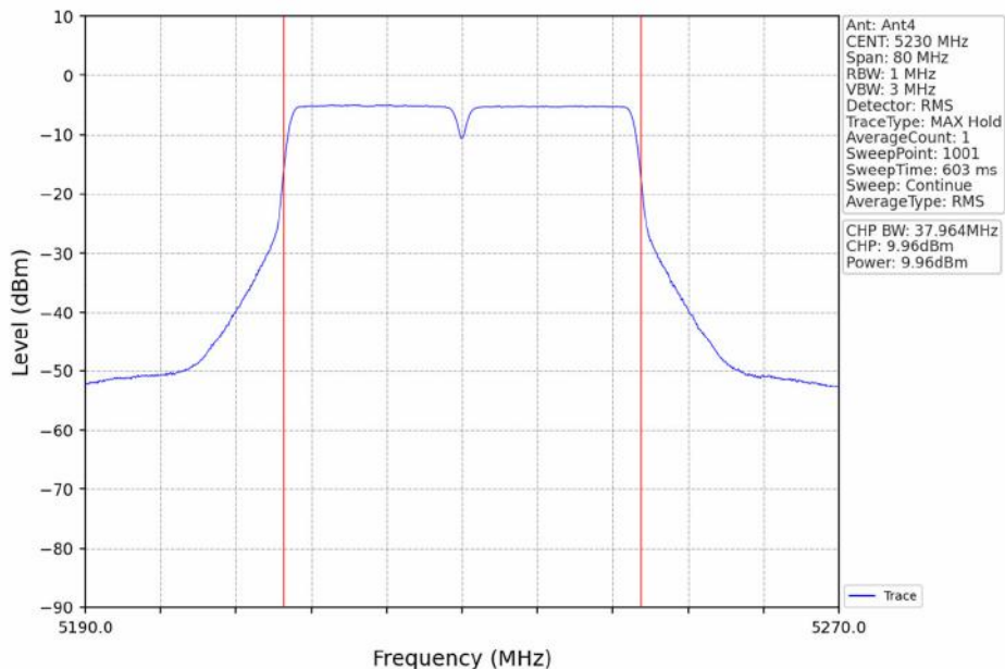
802.11n(HT40)_HCH_5230MHz_Ant4_NTNV
