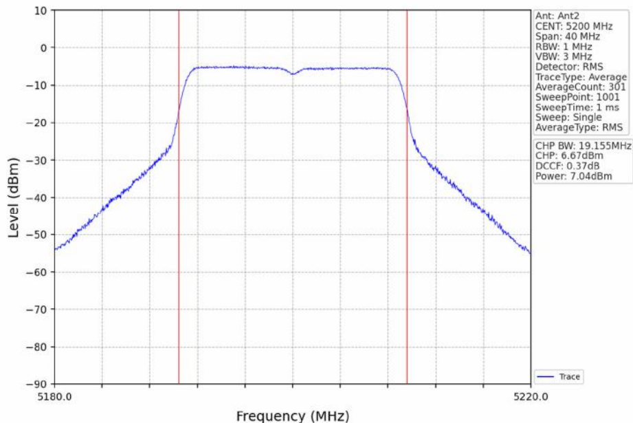
802.11n(HT20)_MCH_5200MHz_Ant2_NTNV
