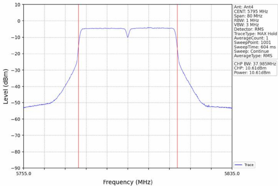
802.11n(HT40)_HCH_5795MHz_Ant4_NTNV
