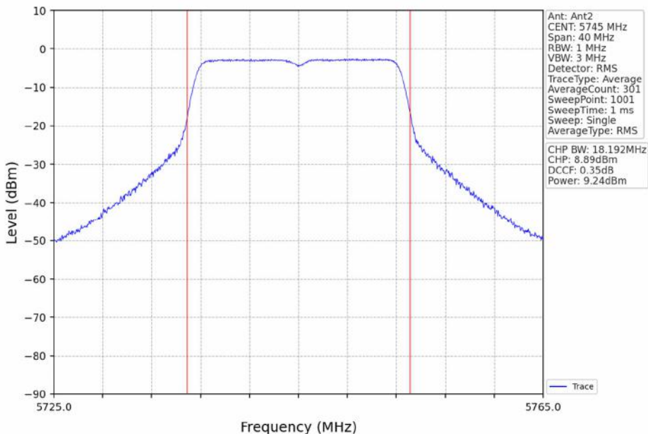
802.11a_LCH_5745MHz_Ant2_NTNV
