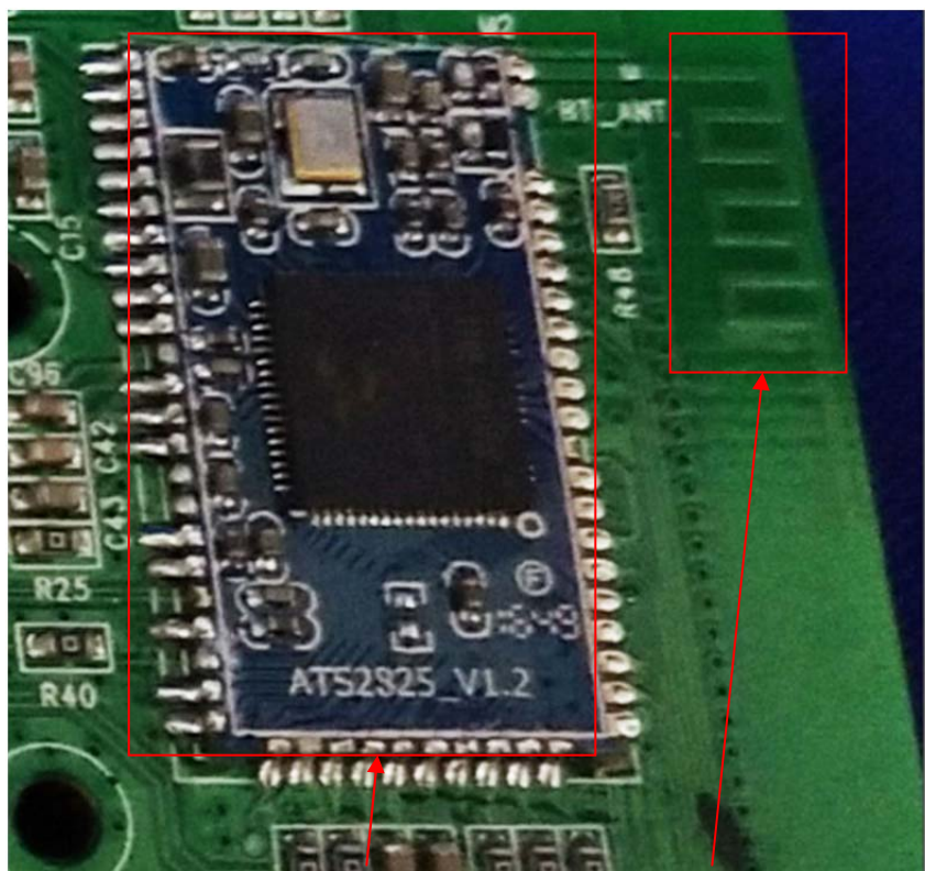
BT module
