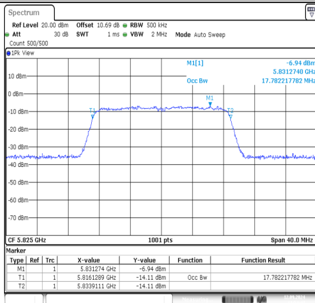
11N20MIMO-Ant1-5825
