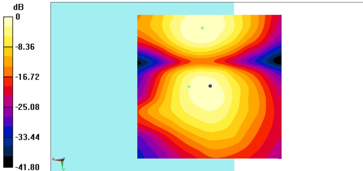
Fig B.1 T-Coil WCDMA850
