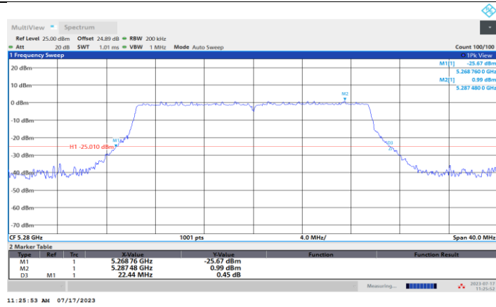
11AX20MIMO_Ant3_5280
