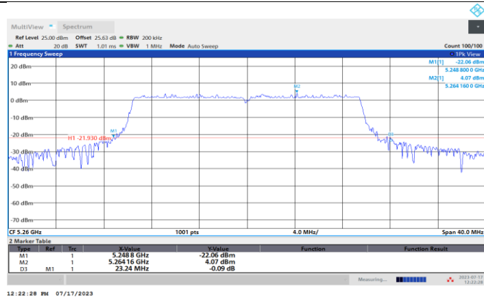
11BE20MIMO_Ant1_5260
