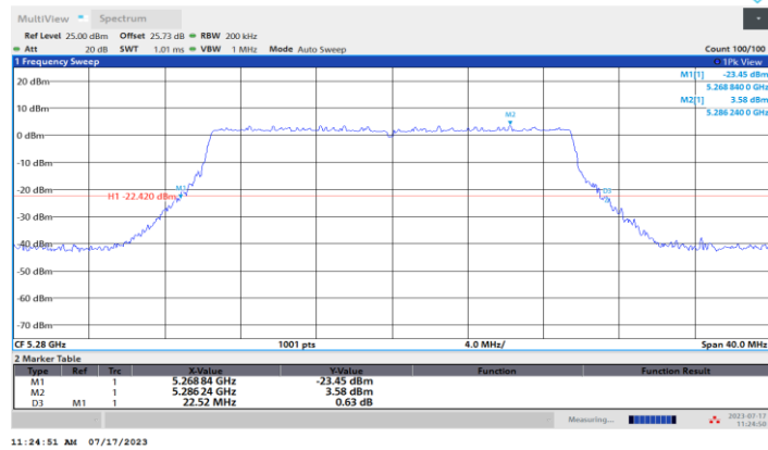
11AX20MIMO_Ant1_5280
