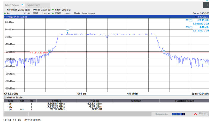
11BE20MIMO_Ant1_5320
