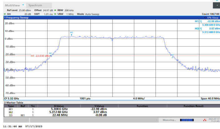
11AX20MIMO_Ant4_5320
