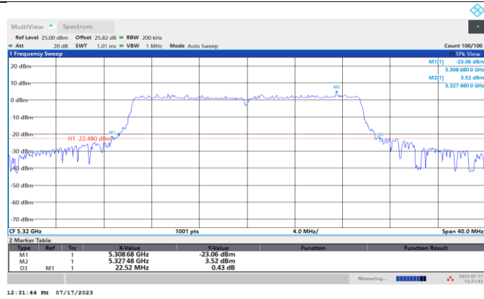
11BE20MIMO_Ant2_5320
