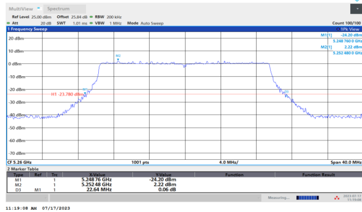
11AX20MIMO_Ant2_5260
