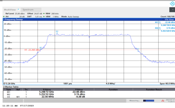
11AX20MIMO_Ant4_5260
