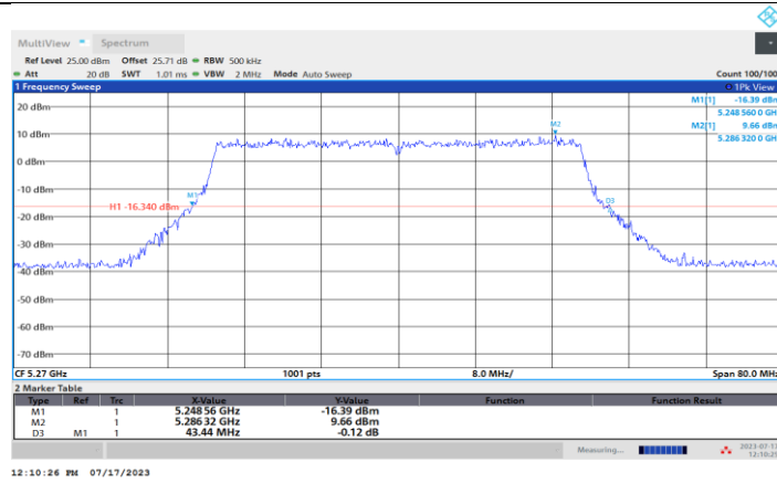
11BE40MIMO_Ant1_5270
