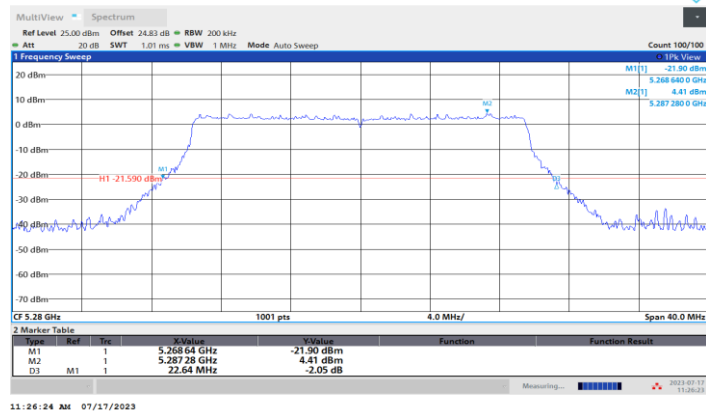
11AX20MIMO_Ant4_5280
