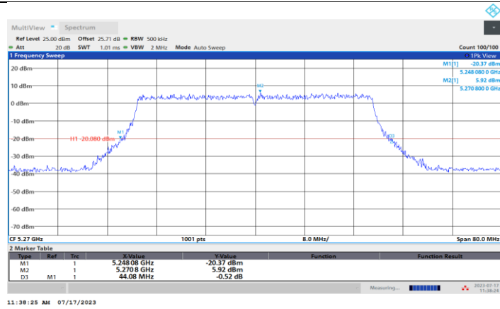
11AX40MIMO_Ant1_5270
