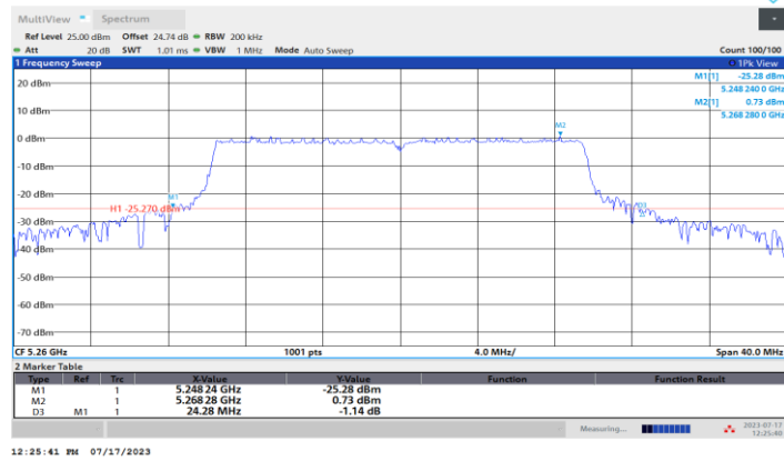
11BE20MIMO_Ant3_5260
