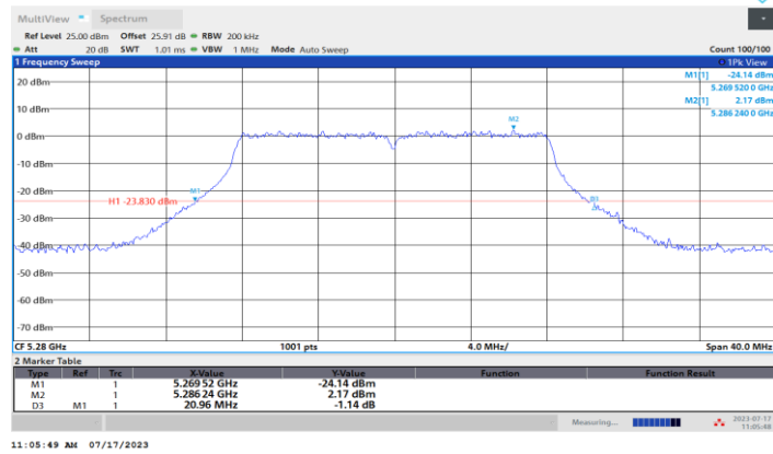
11A-CDD_Ant2_5280
