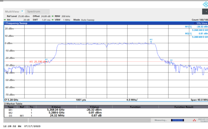
11BE20MIMO_Ant3_5280
