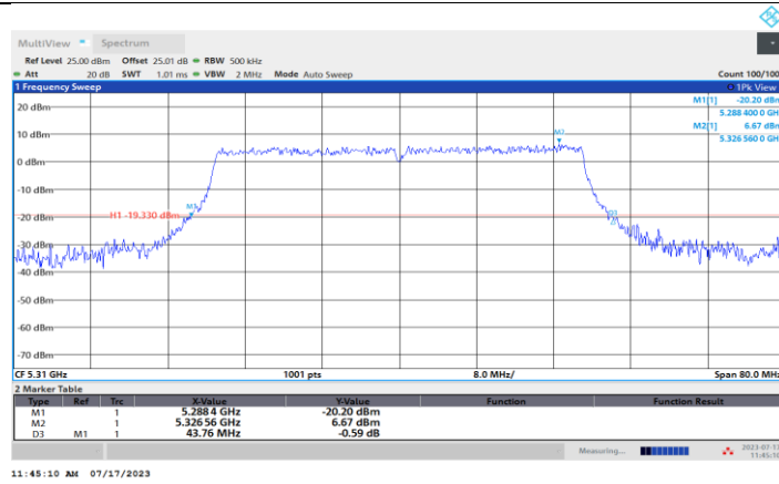
11AX40MIMO_Ant3_5310
