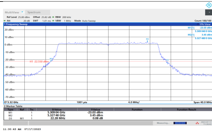
11AX20MIMO_Ant2_5320
