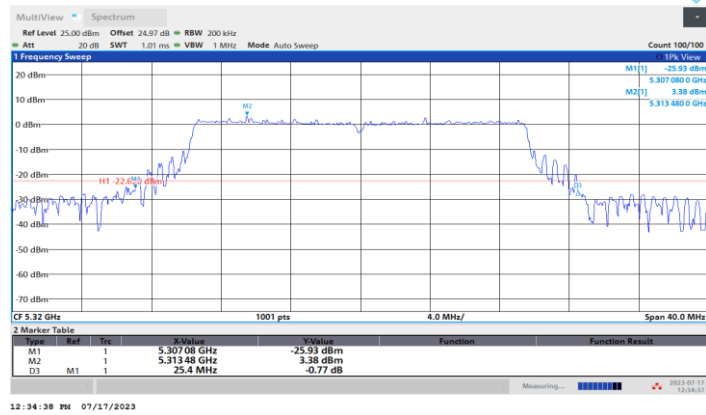
11BE20MIMO_Ant4_5320
