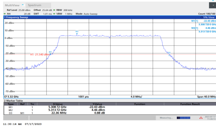
11AX20MIMO_Ant1_5320
