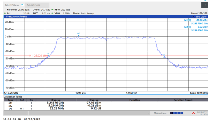
11AX20MIMO_Ant3_5260
