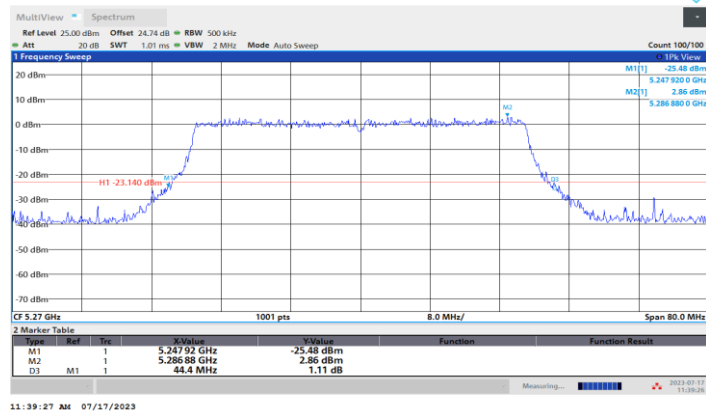
11AX40MIMO_Ant3_5270
