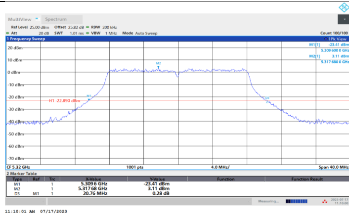
11A-CDD_Ant2_5320
