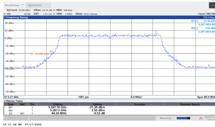
11BE40MIMO_Ant3_5270
