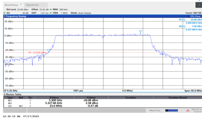
11BE20MIMO_Ant3_5320
