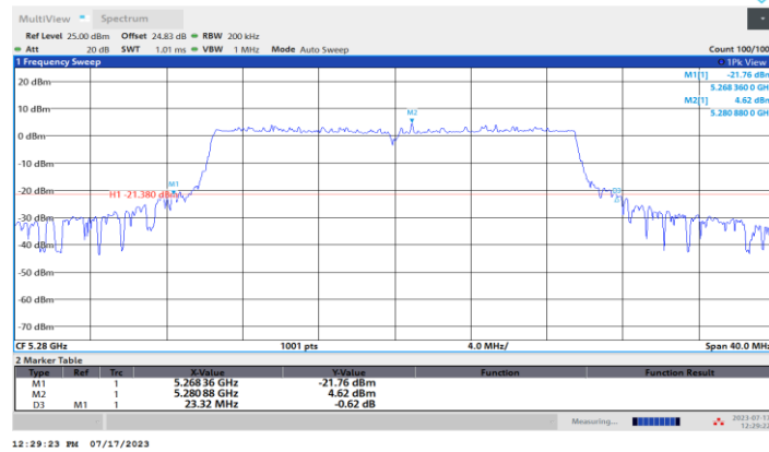
11BE20MIMO_Ant4_5280
