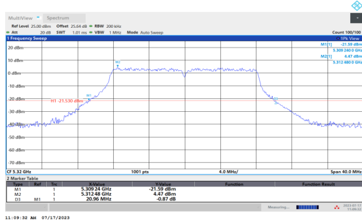
11A-CDD_Ant1_5320
