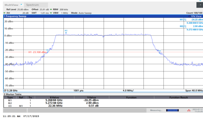
11AX20MIMO_Ant2_5280
