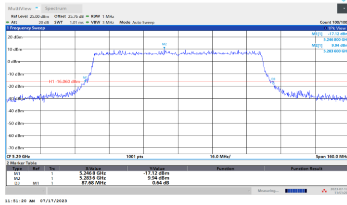
11AX80MIMO_Ant1_5290
