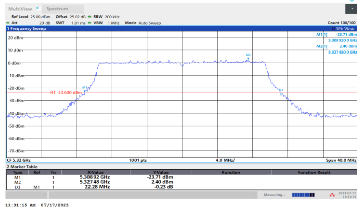
11AX20MIMO_Ant3_5320
