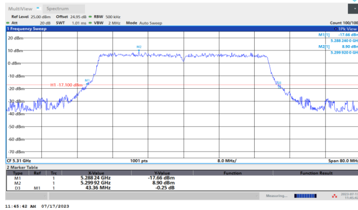
11AX40MIMO_Ant4_5310
