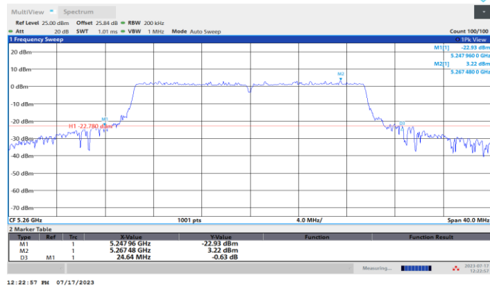
11BE20MIMO_Ant2_5260
