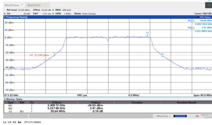
11A-CDD_Ant3_5320
