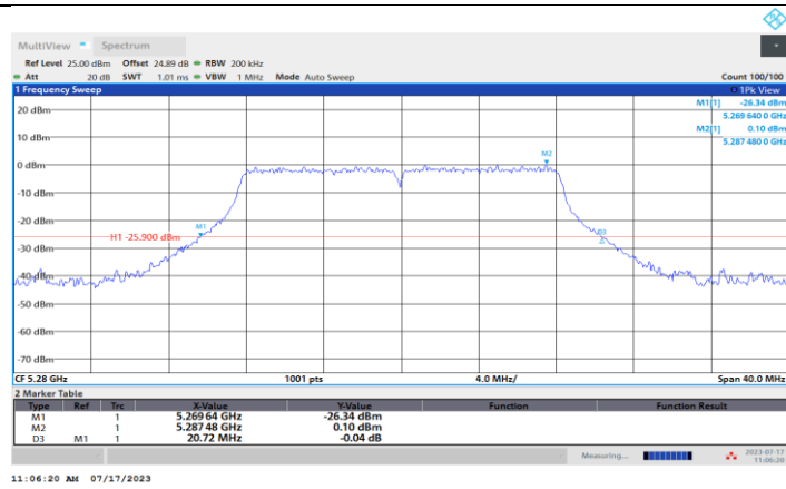
11A-CDD_Ant3_5280
