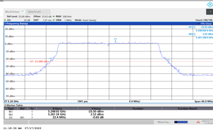
11AX20MIMO_Ant1_5260
