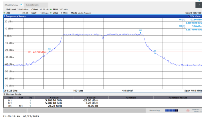
11A-CDD_Ant1_5280
