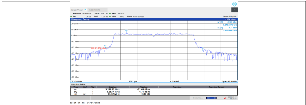
11BE20MIMO_Ant4_5260
