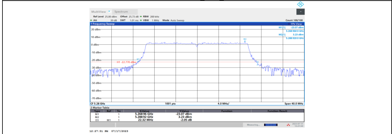
11BE20MIMO_Ant1_5280
