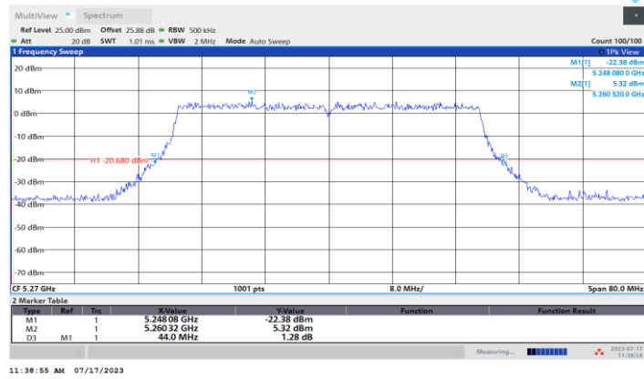
11AX40MIMO_Ant2_5270
