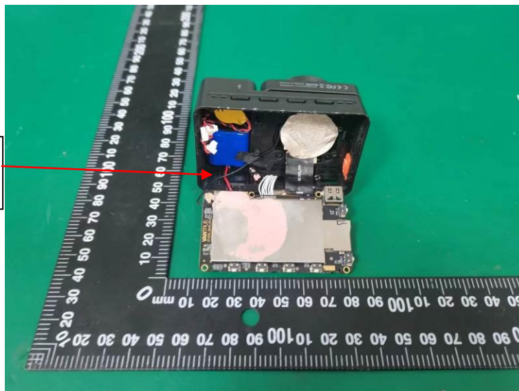
BT&WIFI Antenna
