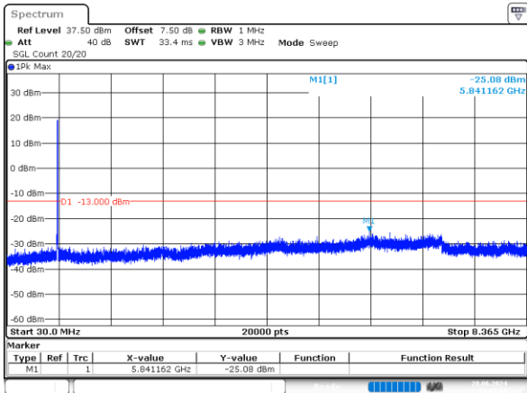
5MHz_Middle_QPSK_25@0 -25.08dBm
