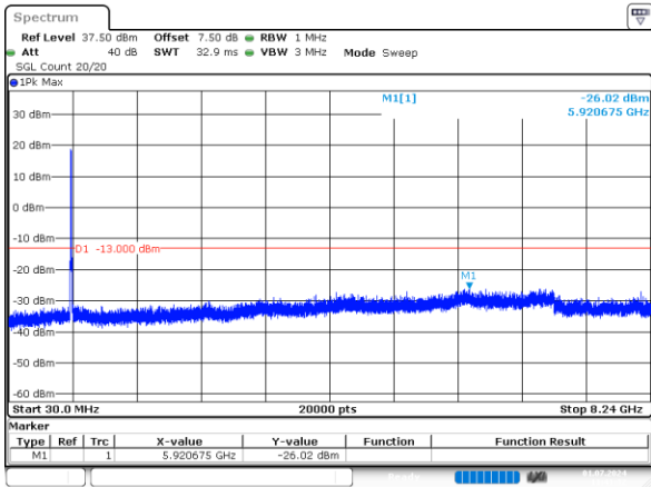
3_10MHz_Middle_QPSK_50@0 -26.02dBm
