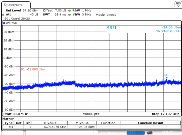
1.4MHz_Low_QPSK_6@0 -24.06dBm
