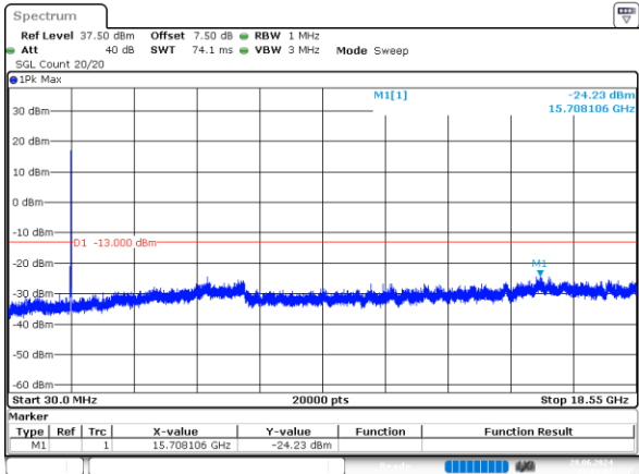
10MHz_Low_QPSK_50@0 -24.23dBm
