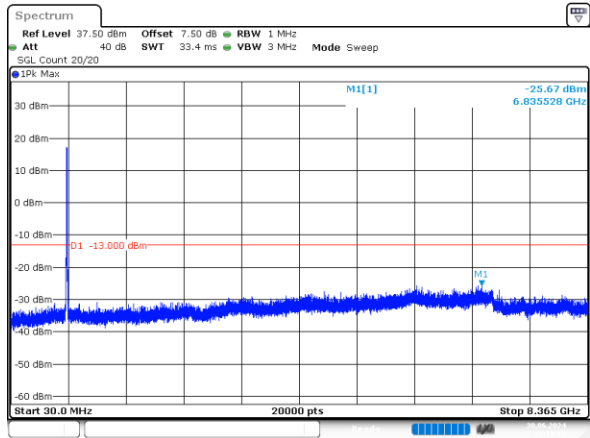
2_10MHz_Middle_QPSK_50@0 -25.67dBm
