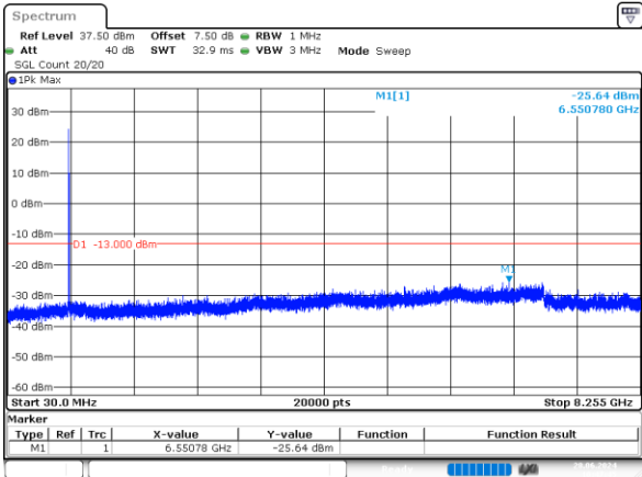
2_3MHz_Low_QPSK_1@0 -25.64dBm
