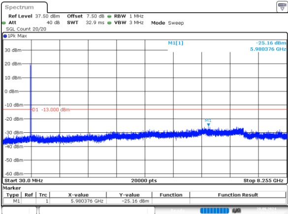
3MHz_Low_QPSK_15@0 -25.16dBm
