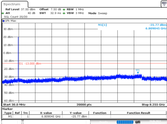
2_3MHz_Low_QPSK_15@0 -25.77dBm
