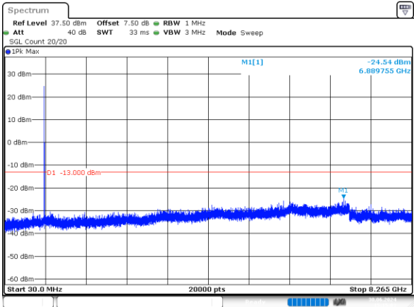
2_5MHz_Low_QPSK_1@0 -24.54dBm
