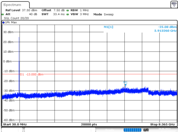
2_5MHz_Middle_QPSK_1@0 -25.08dBm
