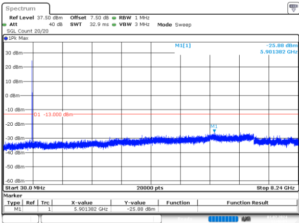
3_3MHz_Middle_QPSK_1@0 -25.88dBm
