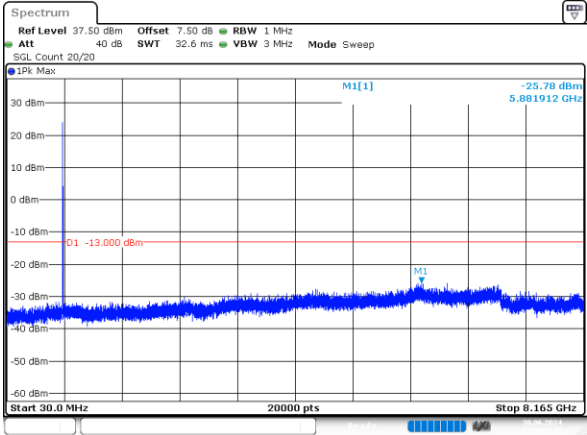
1_5MHz_Low_QPSK_1@0 -25.78dBm
