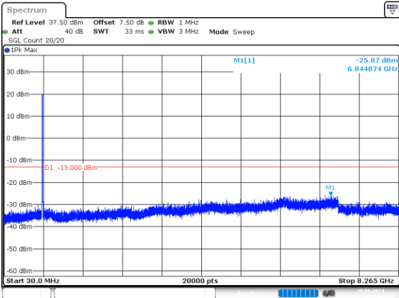
2_5MHz_Low_QPSK_25@0 -25.87dBm
