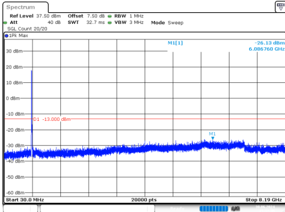
1_10MHz_Middle_QPSK_50@0 -26.13dBm
