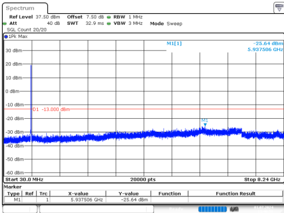
3_5MHz_Middle_QPSK_25@0 -25.64dBm
