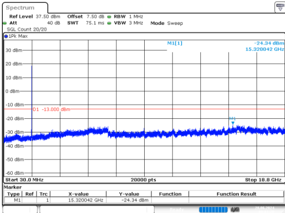
5MHz_Middle_QPSK_25@0 -24.34dBm
