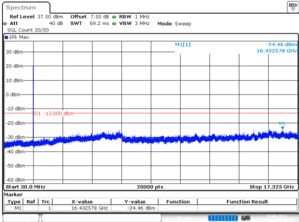
1.4MHz_Middle_QPSK_6@0 -24.46dBm
