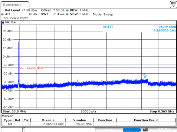
10MHz_Middle_QPSK_50@0 -25.49dBm
