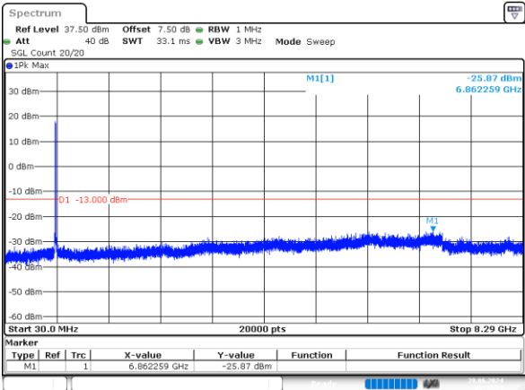
10MHz_Low_QPSK_50@0 -25.87dBm
