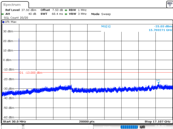
1.4MHz_Low_QPSK_1@0 -25.03dBm
