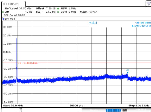
2_15MHz_Low_QPSK_75@0 -25.66dBm
