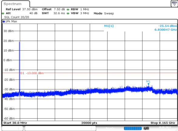
1_5MHz_Low_QPSK_25@0 -25.54dBm
