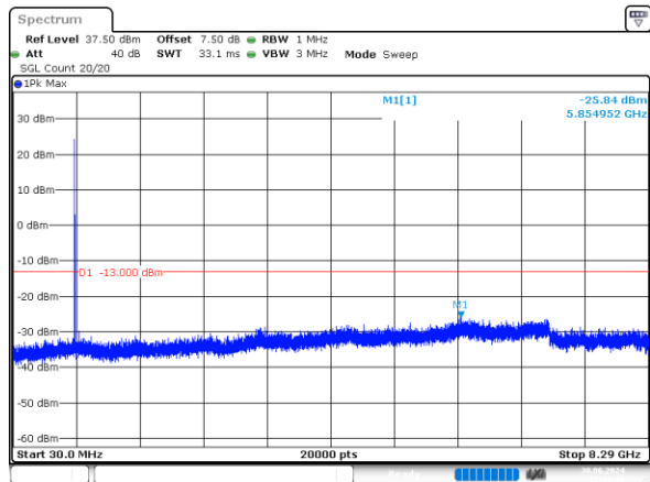
2_10MHz_Low_QPSK_1@0 -25.84dBm
