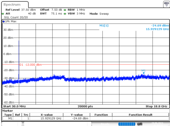
10MHz_Middle_QPSK_50@0 -24.69dBm
