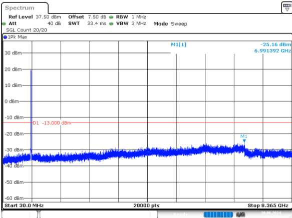
2_5MHz_Middle_QPSK_25@0 -25.16dBm
