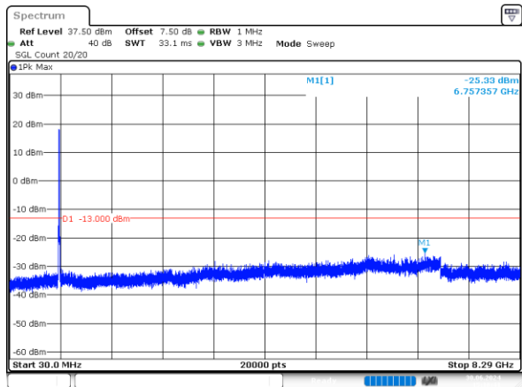
2_10MHz_Low_QPSK_50@0 -25.33dBm
