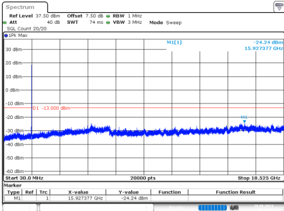
5MHz_Low_QPSK_25@0 -24.24dBm
