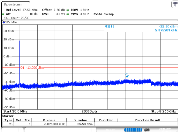
5MHz_Low_QPSK_25@0 -25.50dBm
