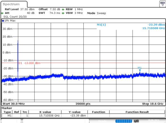
20MHz_Low_QPSK_100@0 -23.39dBm
