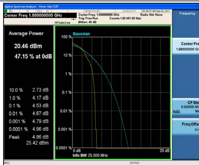
Band2_15MHz_QPSK_18900_75RB#0_4.52_13_PASS
