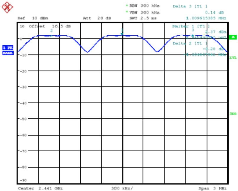
(Plot B: \pi/4 -DQPSK Channel)
