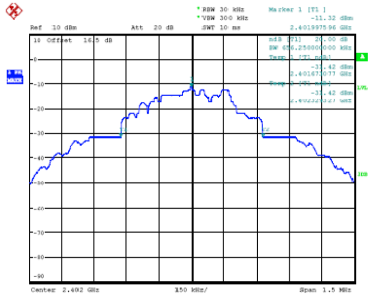
(Plot A: Channel = 2402)
