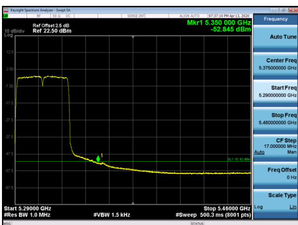
5310MHz with 2*2 CDD AV
