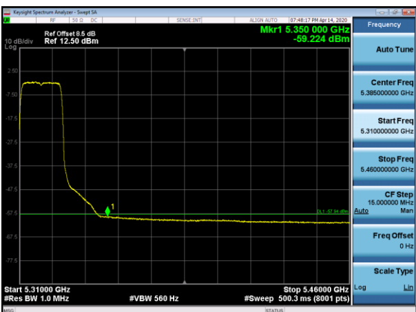
5320MHz with 4*4 CDD AV
