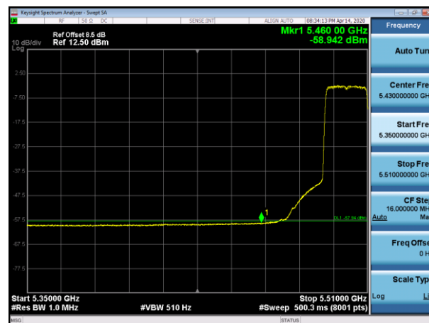
5500MHz with 4*4 CDD AV
