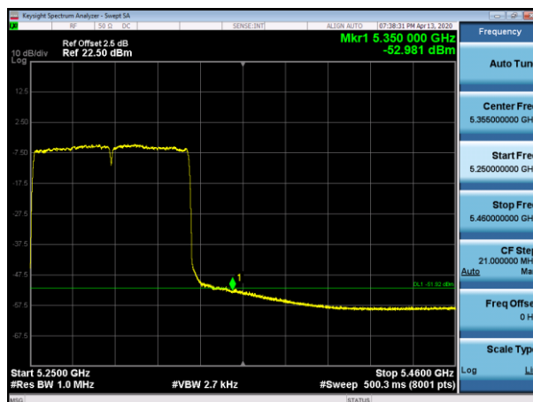
5290MHz with 2*2 CDD AV
