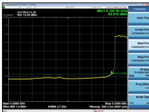
5210MHz with 2*2 CDD AV
