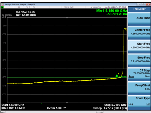
5200MHz with 4*4 CDD AV
