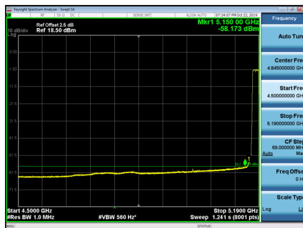
5180MHz with 4*4 CDD AV
