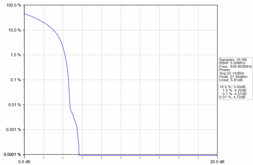
Band5_HSUPA_MCH_836.6MHz_Subtest 1_NTNV
