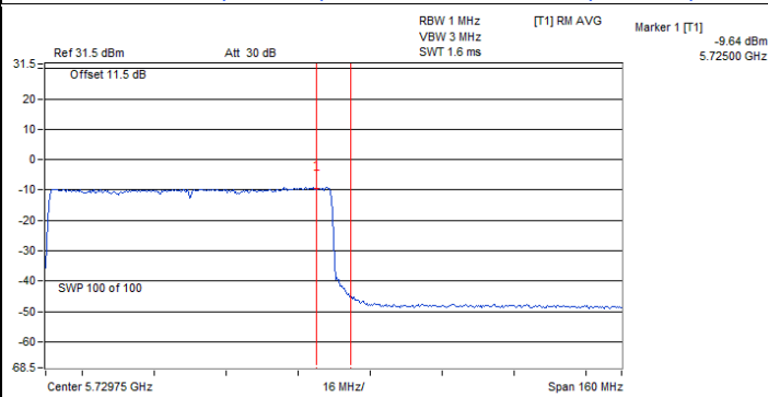
802.11be (EHT80) / Chain 0 : CH 138 (U-NII-3)
