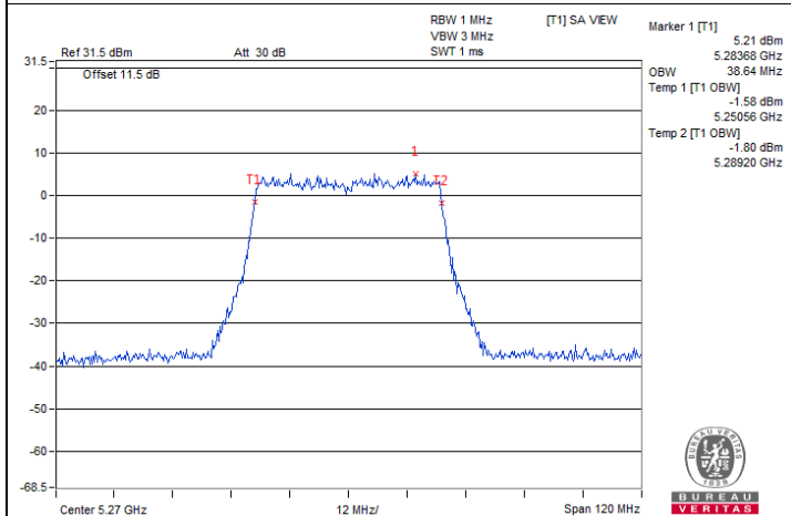
802.11be (EHT40) / Chain 0 : CH 54
