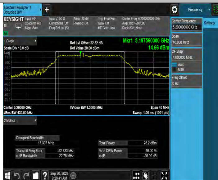
11A-MIMO_Ant3_5200
