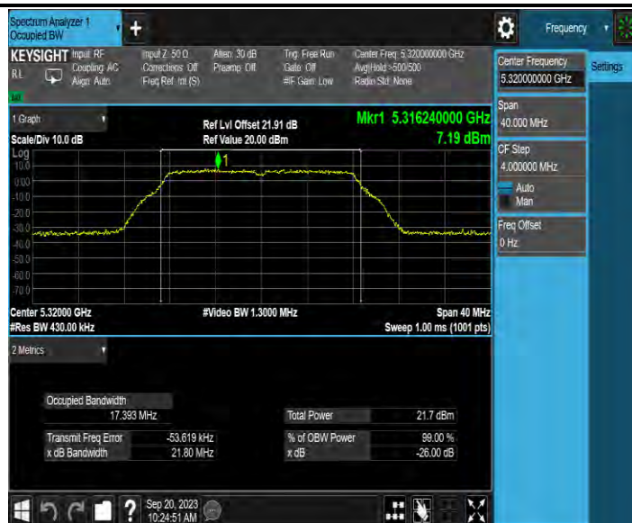
11A-MIMO_Ant4_5320
