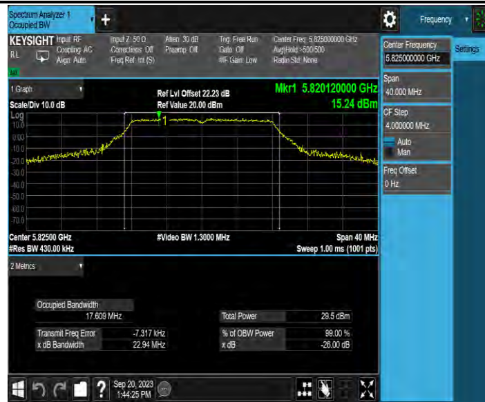
11A-MIMO_Ant4_5825
