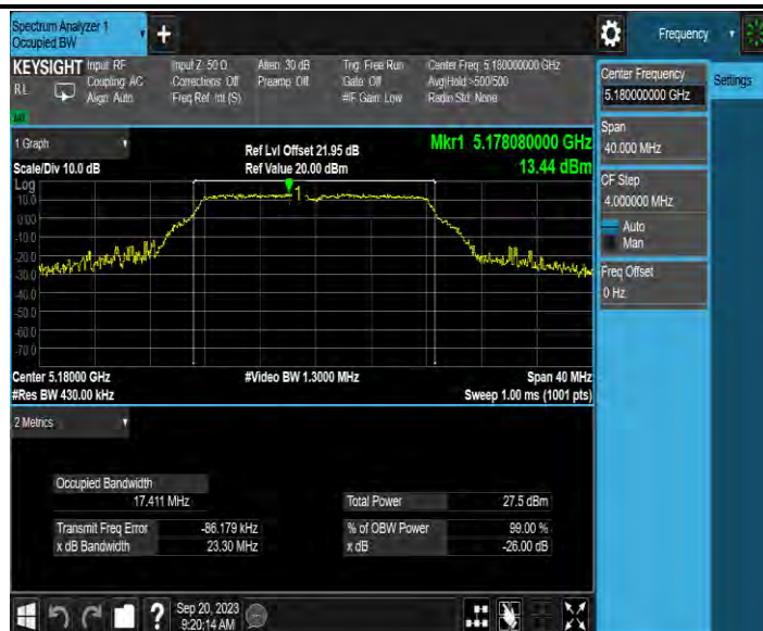
11A-MIMO_Ant4_5180
