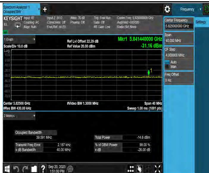
11A-MIMO_Ant2_5825
