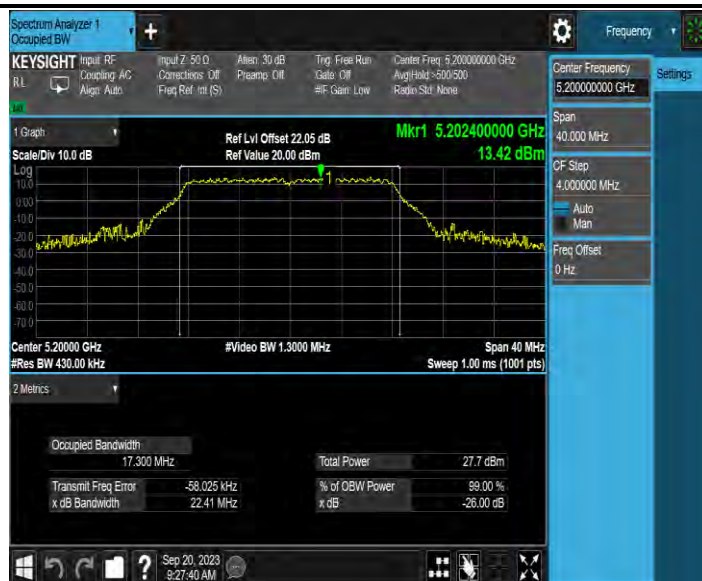
11A-MIMO_Ant2_5200
