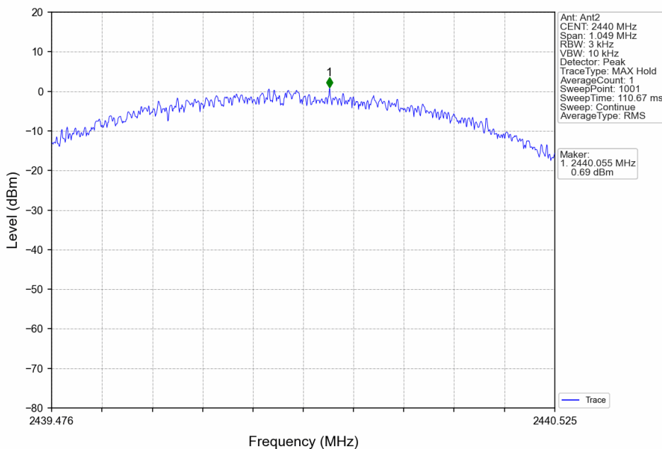
1M_MCH_2440MHz_Ant2_NTNV
