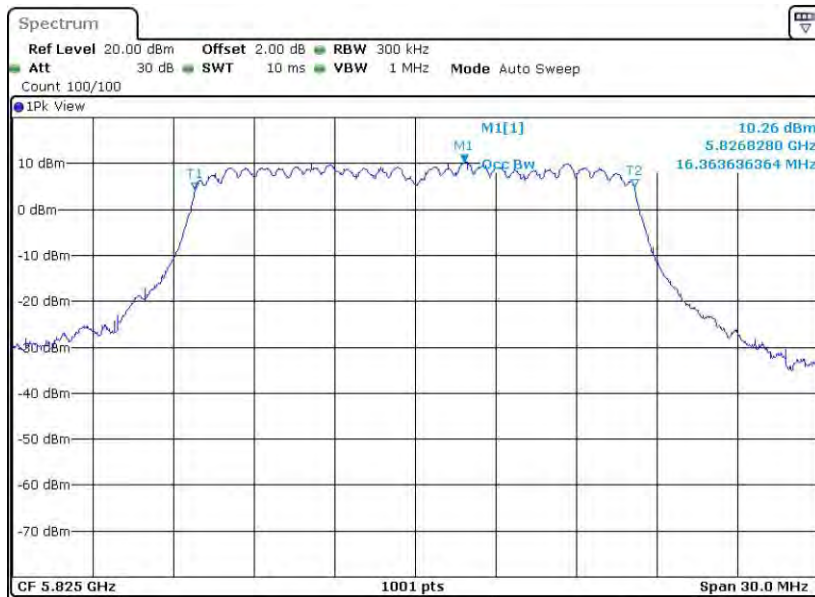
11A-CDD_Ant1_5825
