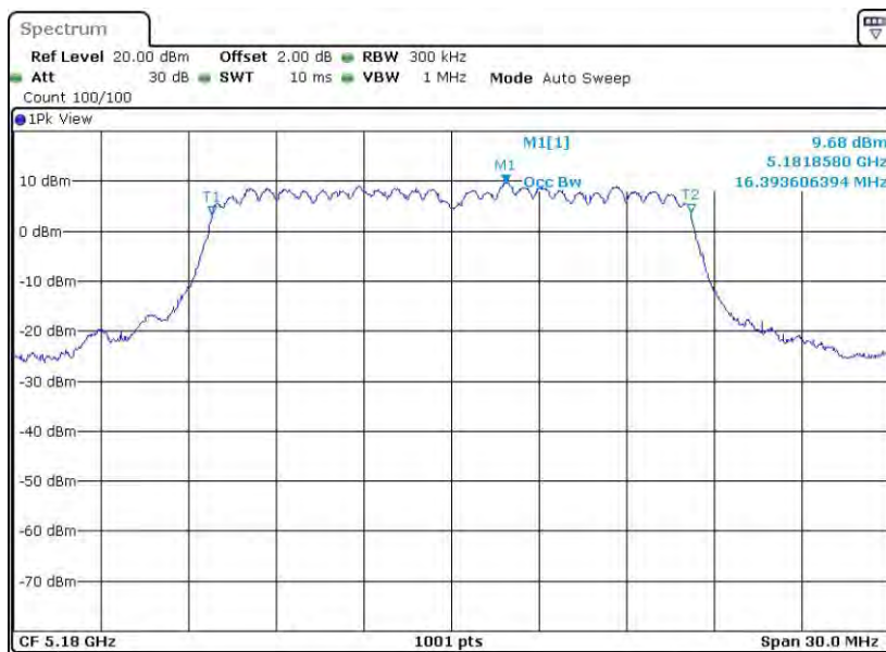
11A-CDD_Ant2_5180
