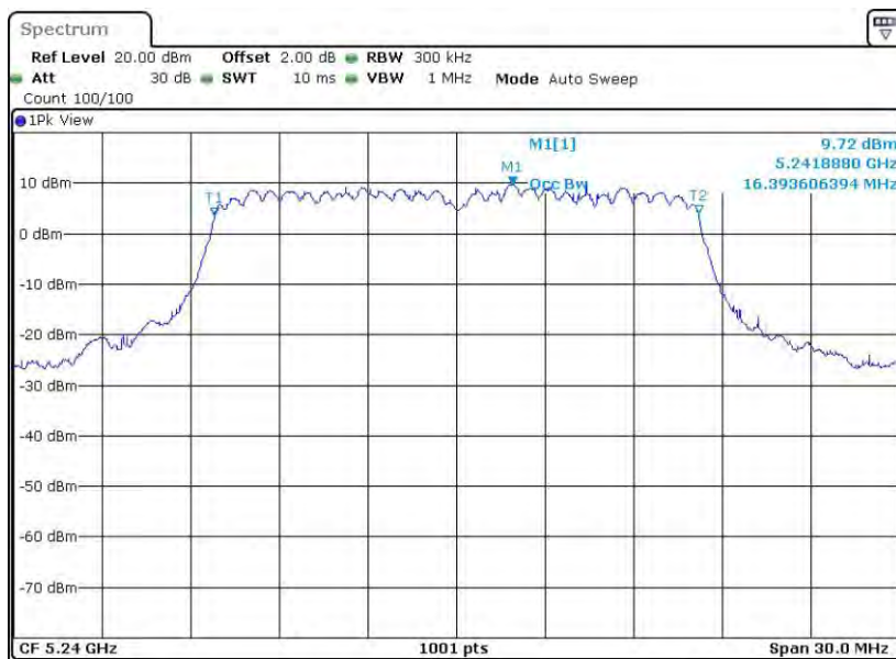
11A-CDD_Ant2_5240
