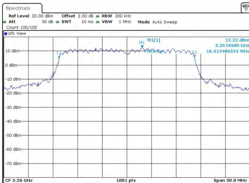
11A-CDD_Ant1_5260
