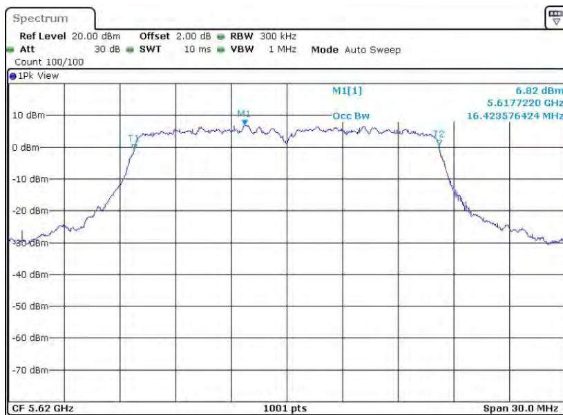
11A-CDD_Ant2_5620
