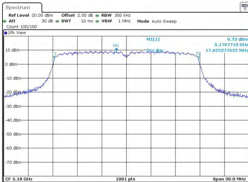
11N20MIMO_Ant2_5180
