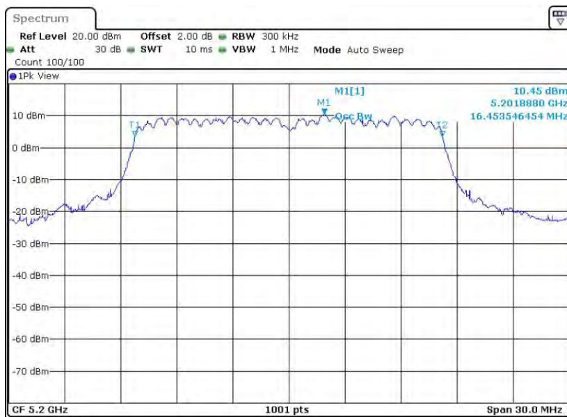
11A-CDD_Ant1_5200
