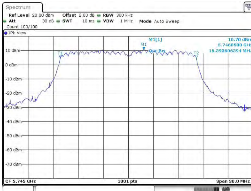
11A-CDD_Ant1_5745
