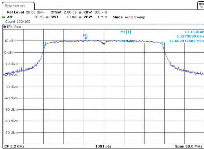
11N20MIMO_Ant1_5200
