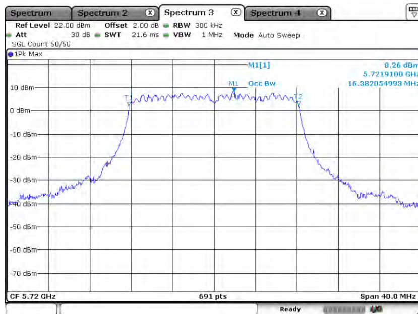
11A-CDD_Ant2_5720
