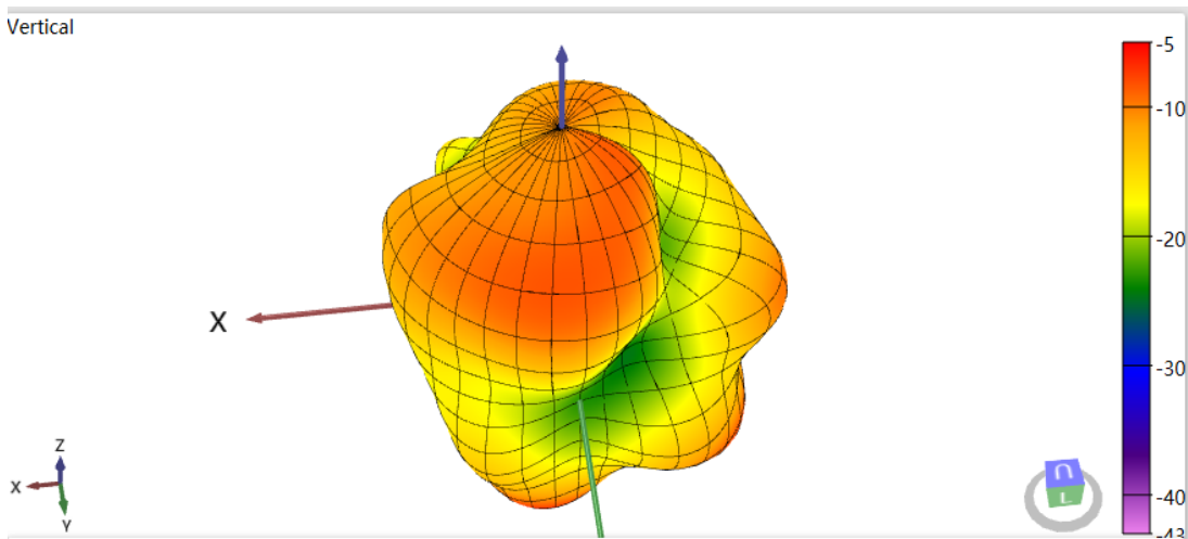
天线 2440MHz 3D-Vertical Pattern
