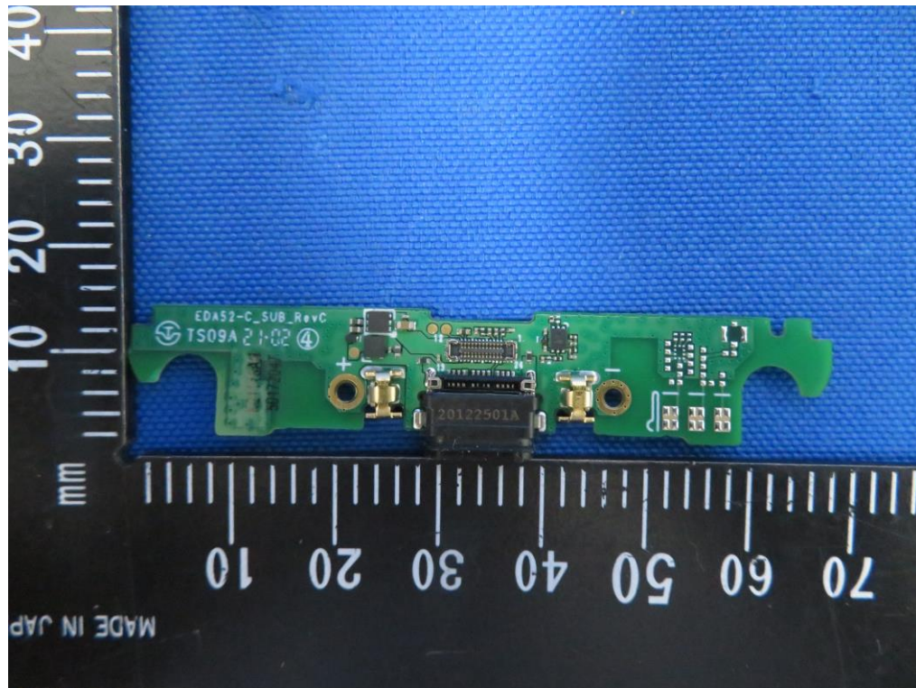
(30) EUT Photo
