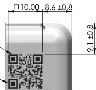
DÉTAIL C ECHELLE 3 : 2
