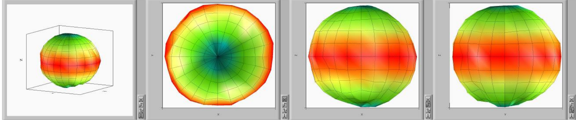
5850MHz Total
