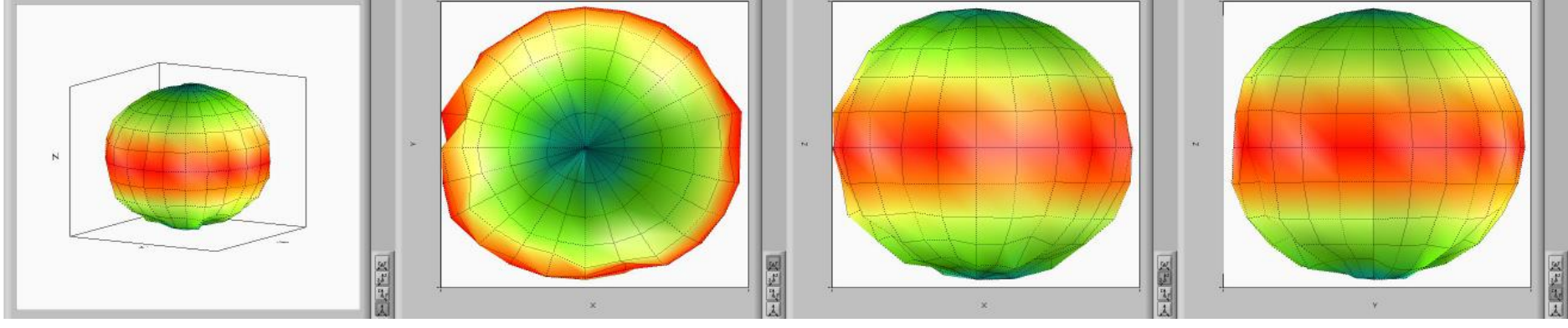
7200MHz Total
