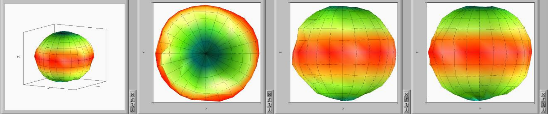
5150MHz Total
