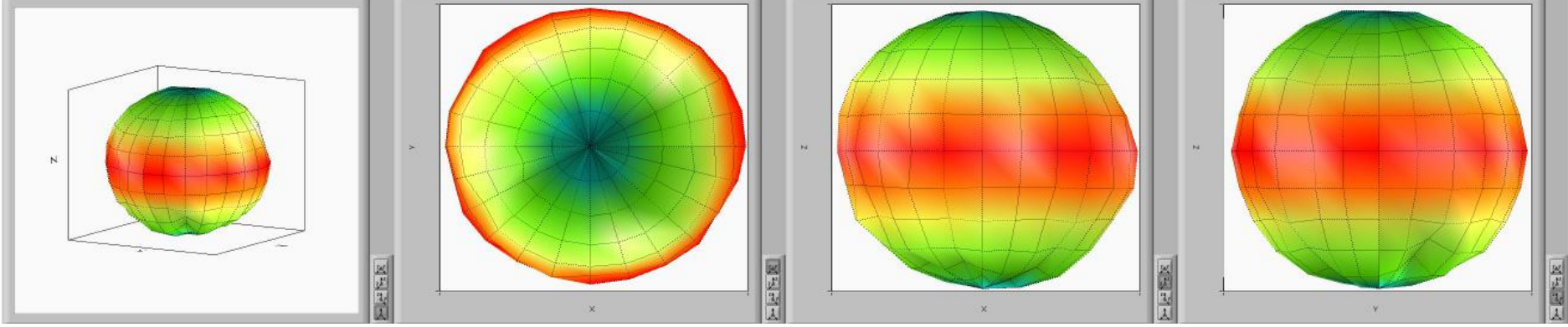
6900MHz Total
