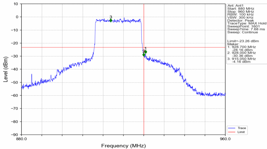
20M_HCH_918MHz_Ant1_NTNV
