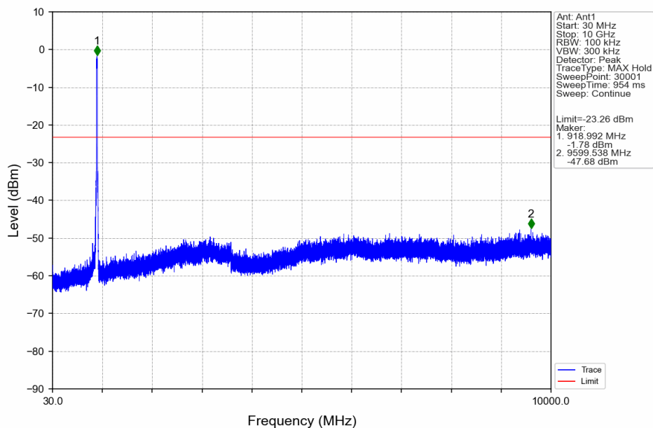
20M_HCH_918MHz_Ant1_NTNV
