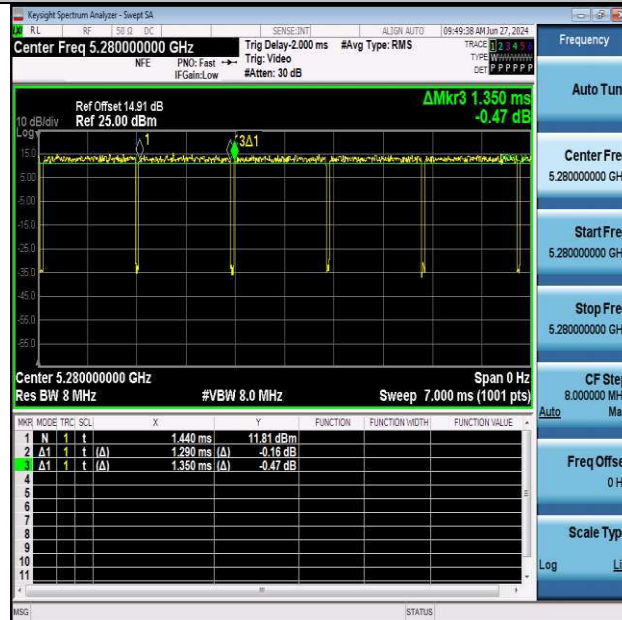
NTNV-11N20MIMO-Ant2-5280
