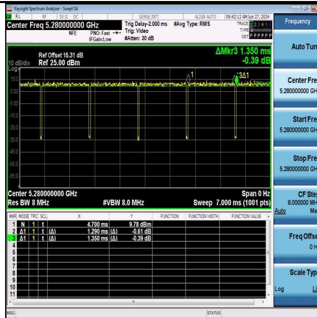
NTNV-11N20MIMO-Ant1-5280
