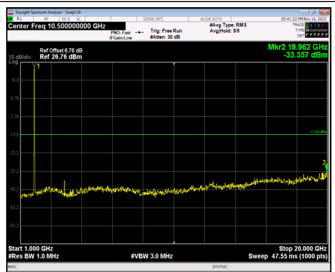
Band2-20MHz-QPSK-19100-1RB#0-Range2:1000~2 0000MHz
