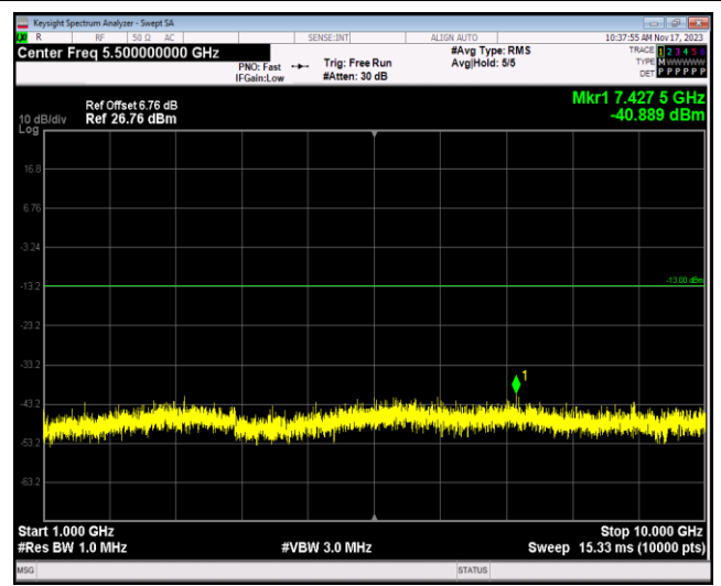
Band13-5MHz-QPSK-23230-1RB#0-Range2:1000~1 0000MHz
