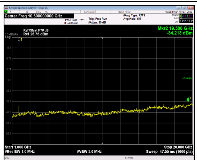
Band4-20MHz-QPSK-20050-1RB#0-Range2:1000~2 0000MHz
