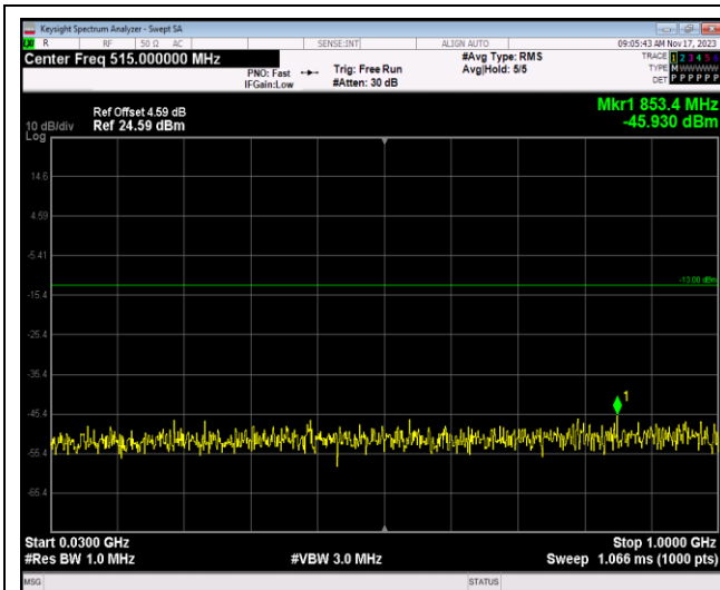
Band4-20MHz-QPSK-20050-1RB#0-Range1:30~100 OMHz
