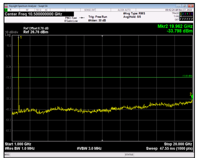
Band4-20MHz-QPSK-20175-1RB#0-Range2:1000~2 0000MHz
