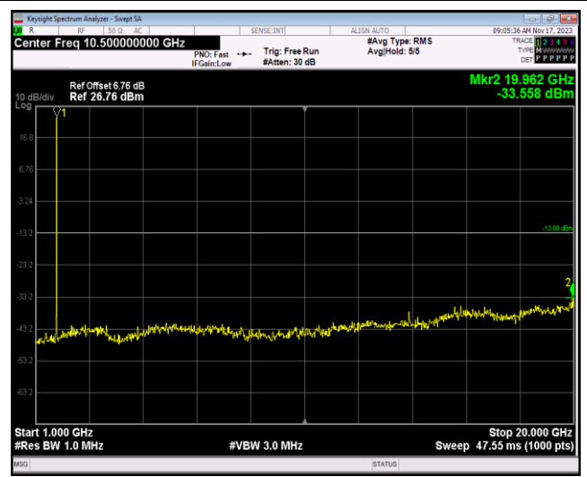
Band4-1.4MHz-QPSK-20393-1RB#0-Range2:1000~20000MHz
