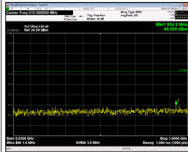
Band4-1.4MHz-QPSK-20393-1RB#0-Range1:30~1000MHz
