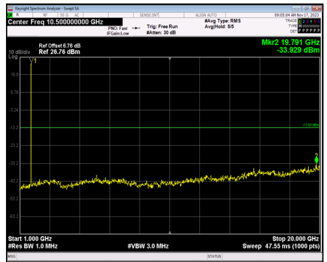
Band4-1.4MHz-QPSK-20393-1RB#0-Range2:1000~20000MHz
