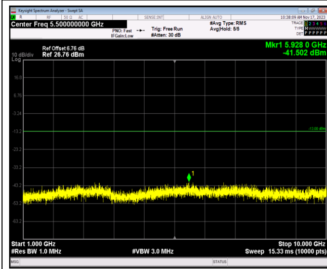
Band13-5MHz-QPSK-23230-1RB#0-Range4:1000~1 0000MHz
