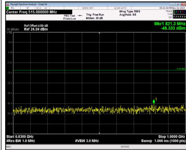
Band2-20MHz-16QAM-18700-1RB#0-Range1:30~10 00MHz
