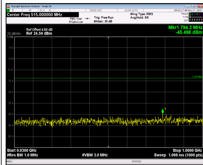
Band4-20MHz-QPSK-20175-1RB#0-Range1:30~100 OMHz
