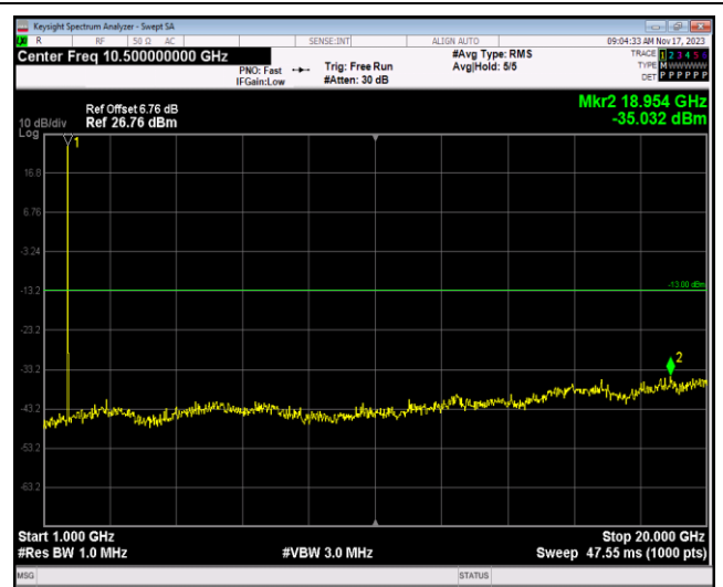
Band4-1.4MHz-QPSK-20175-1RB#0-Range2:1000~20000MHz
