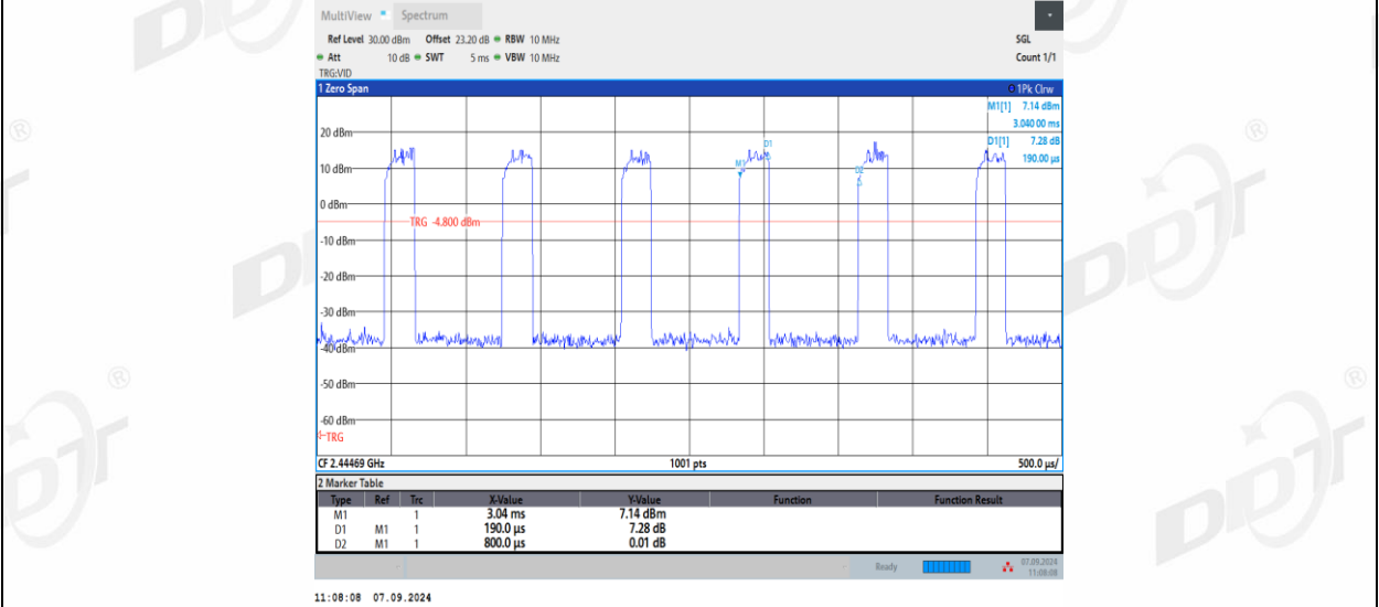
11AX20MIMO_Ant2_2437_26Tone_RU0
