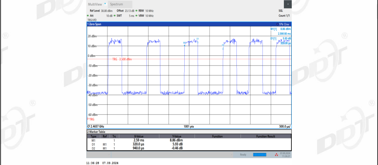
11AX20MIMO_Ant2_2462_52Tone_RU40
