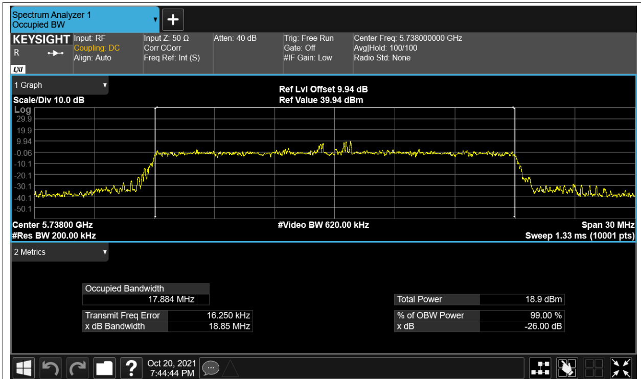
OBW HVHT 5.8G-20M-16QAM 5738MHz Ant2
